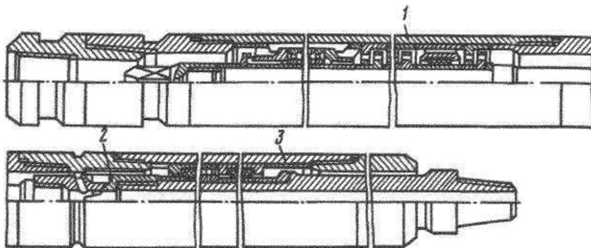
Рисунок 25 – Турбинный отклонитель ТО2:
