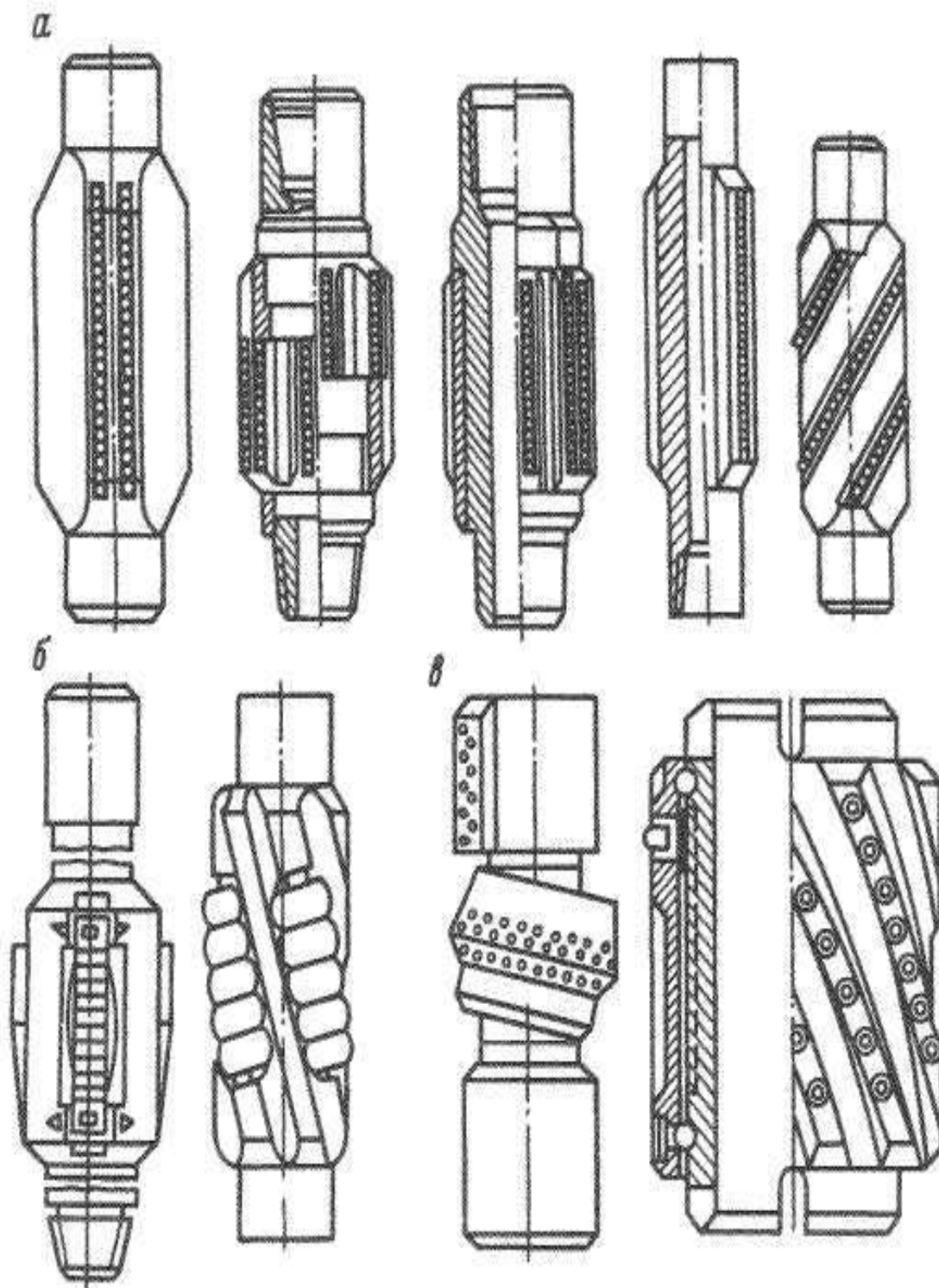
Рисунок 29 – Калибраторы:
