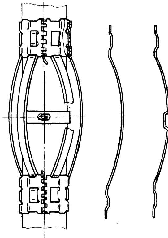
Рисунок 37 - Центратор типа ЦЦ
