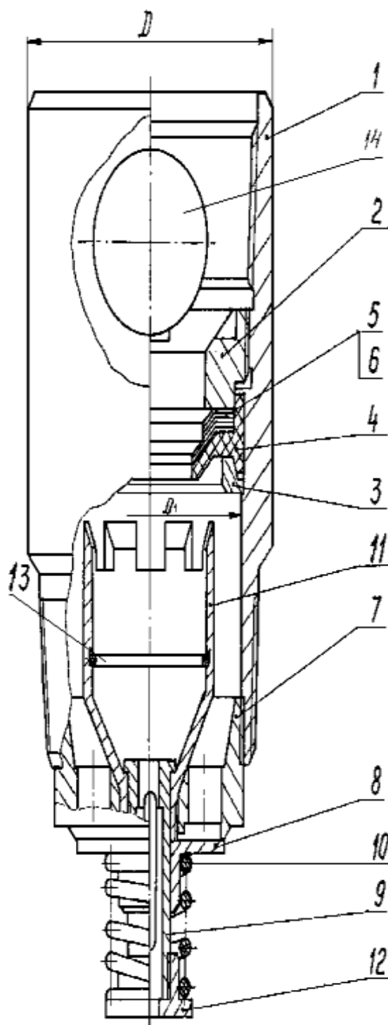
Рисунок 34 - Клапан обратный дроссельный
