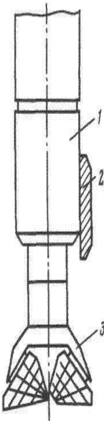
Рисунок 26 – Эксцентричный ниппель:
