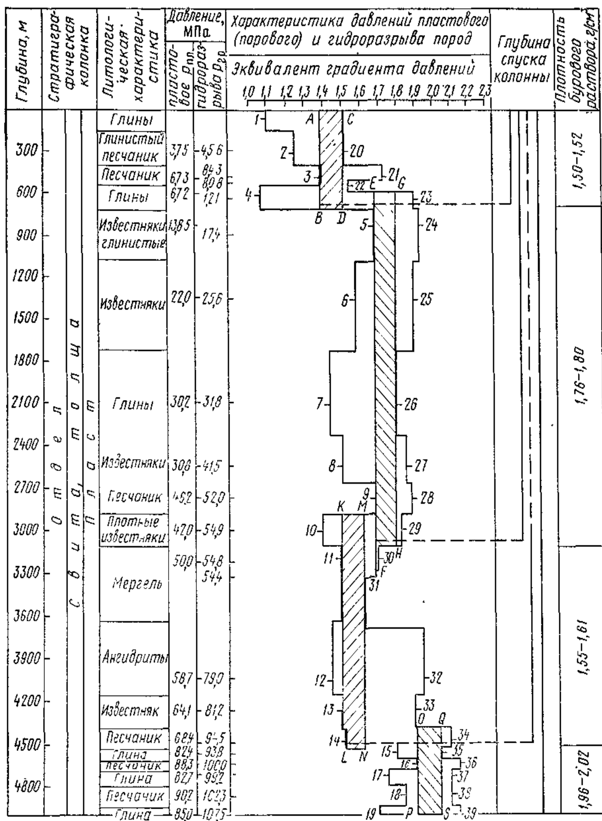
Рисунок 32 – Совмещенный график давлений для выбора конструкции скважины
