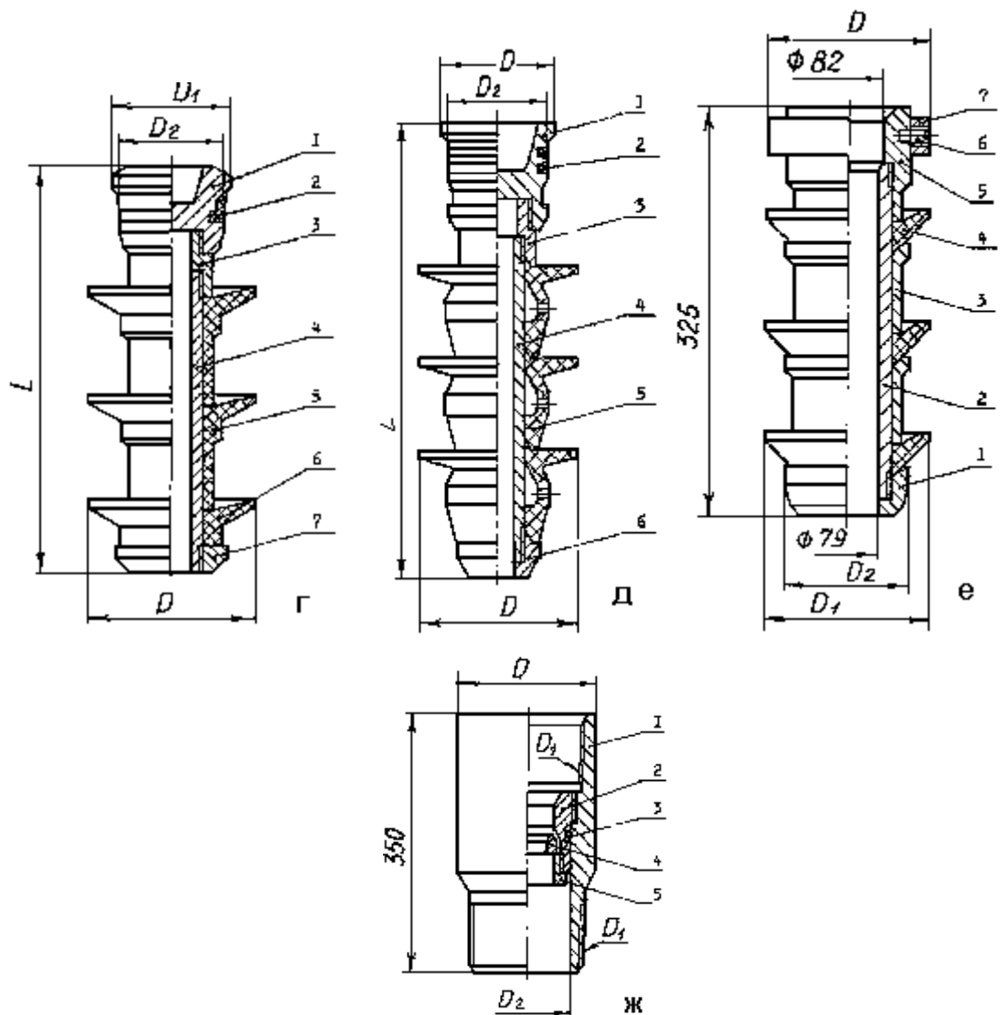
Рисунок 41 - Разновидности ПДМ:
