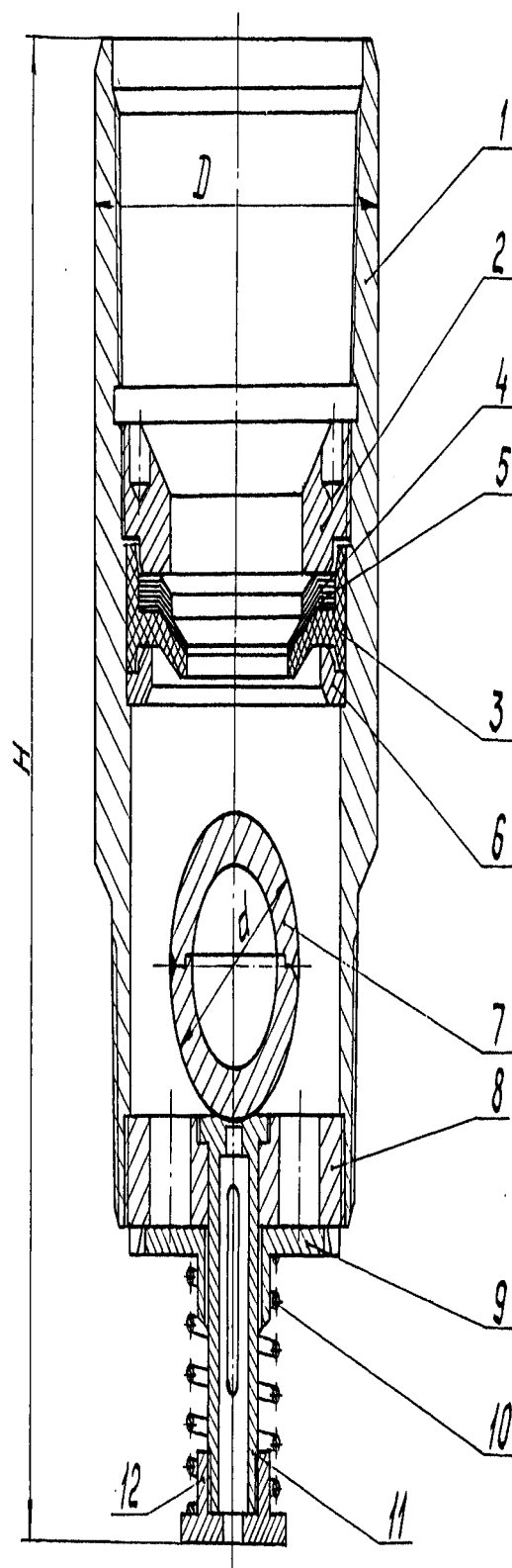
Рисунок 35 - Клапан обратный дроссельный модернизированный ЦКОДМ:
