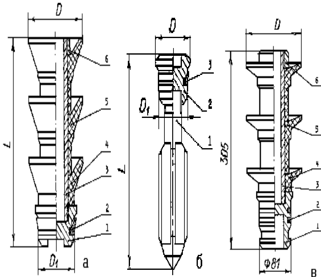
Рисунок 40- Пакер проходной гидравлический универсальный за колонный типа ППГУ:
