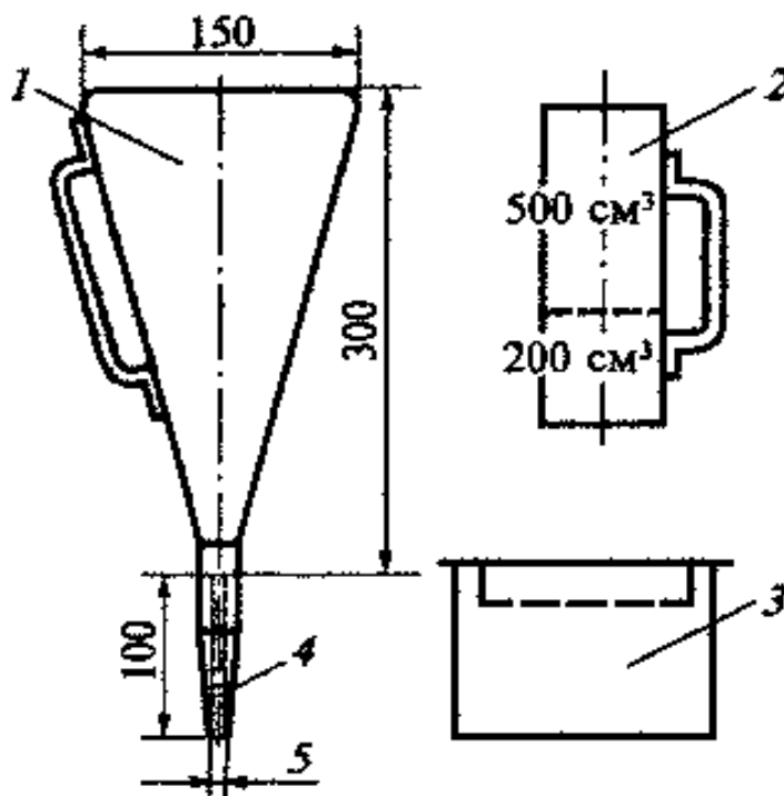
Рисунок 11 – Вискозиметр СПВ–5
