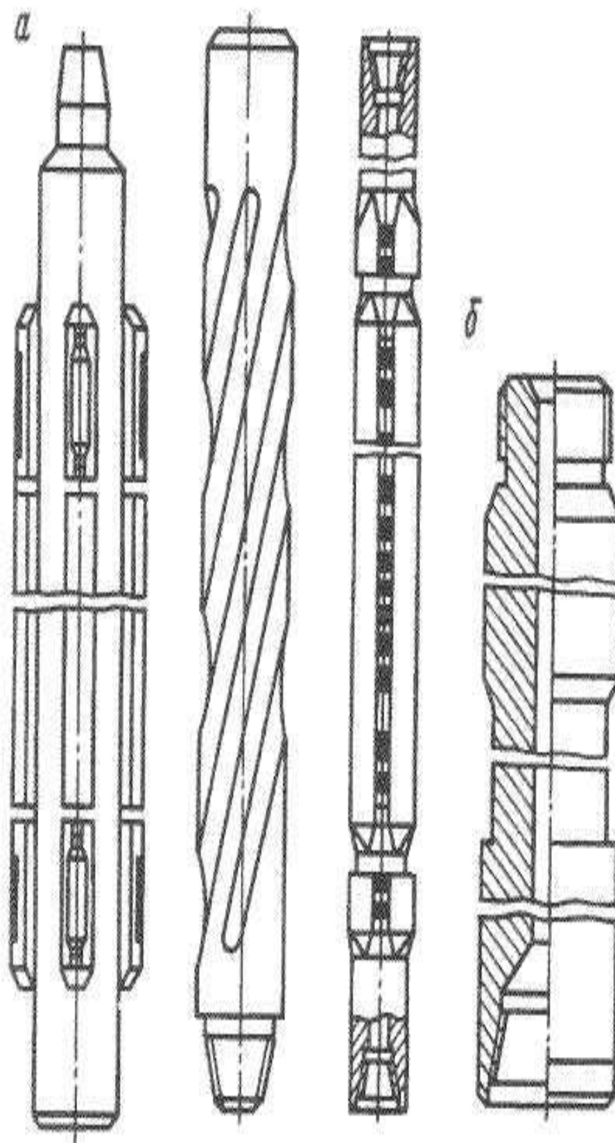
Рисунок 31 – Стабилизирующие устройства:
