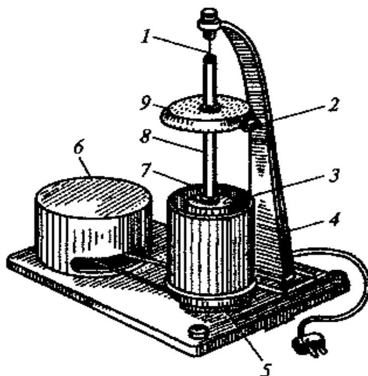
Рисунок 15 – Прибор СНС-2
