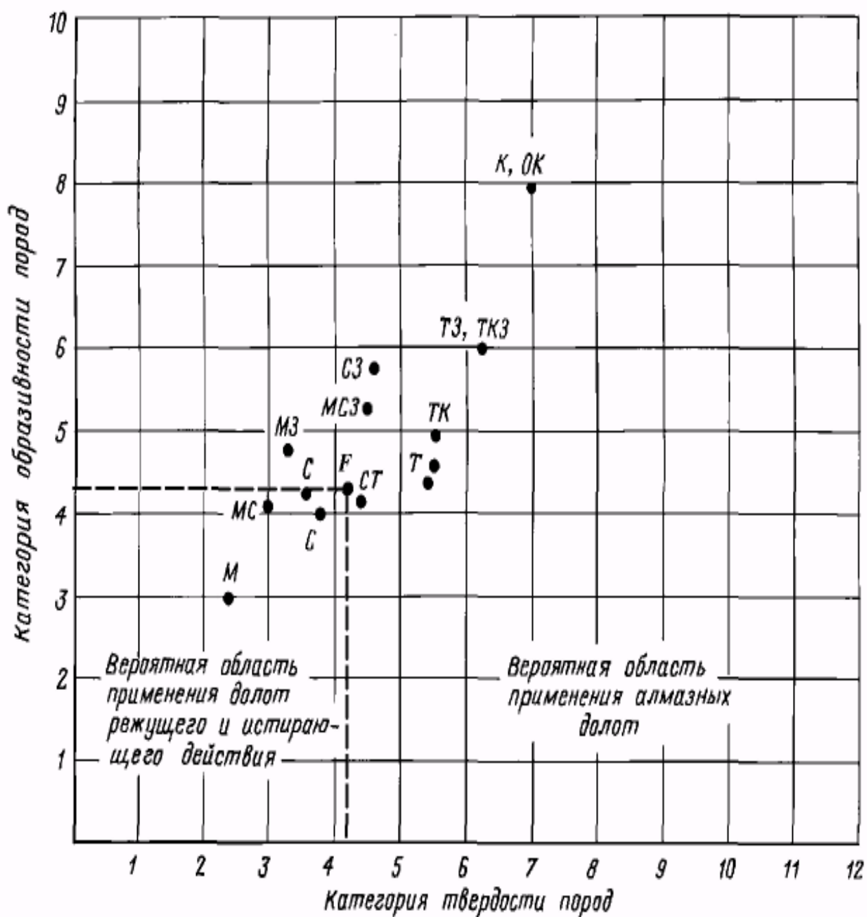
Рисунок 9 – Классификационная таблица парных соответствий категорий твердости и абразивности пород типам шарошечных долот
