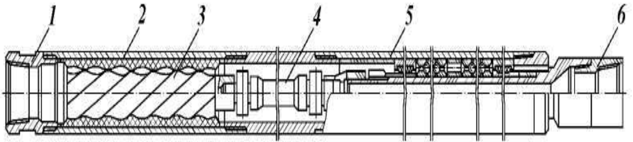
Рисунок 22 – Винтовой забойный двигатель типа Д:
