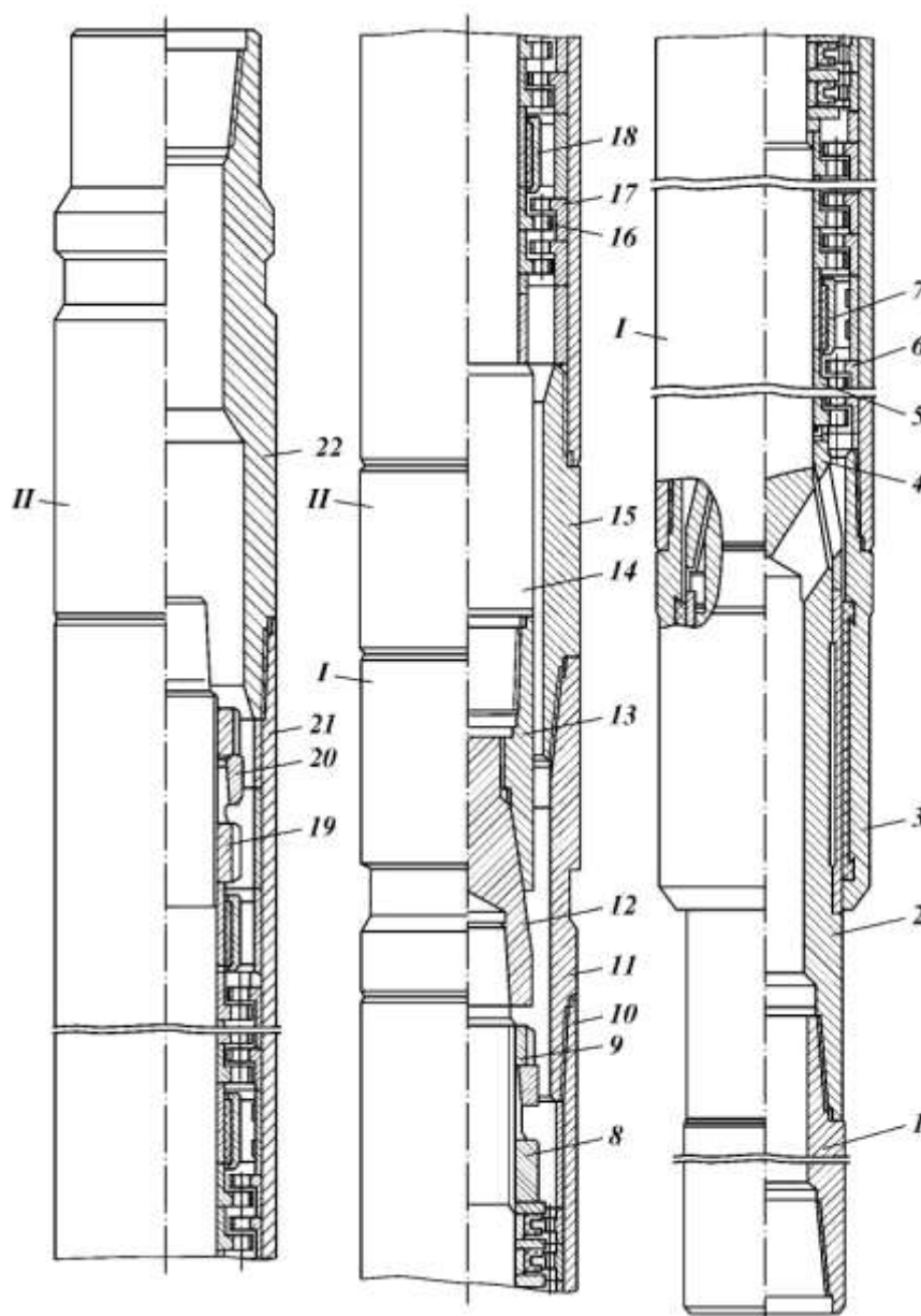
Рисунок 20 – Турбобур секционный бесшпиндельный типа ТС (ТС5Б-240):
