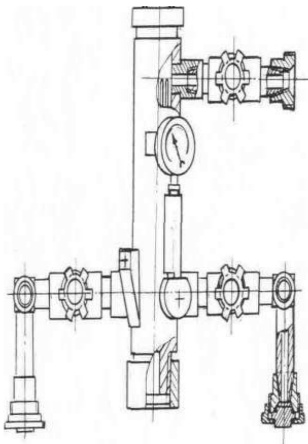
Рисунок 36 - Головка цементирующая
