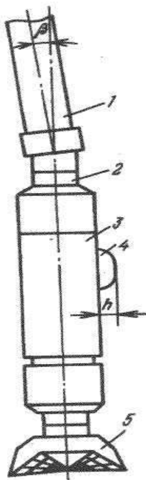
Рисунок 24 – Отклоняющее устройство с накладкой:
