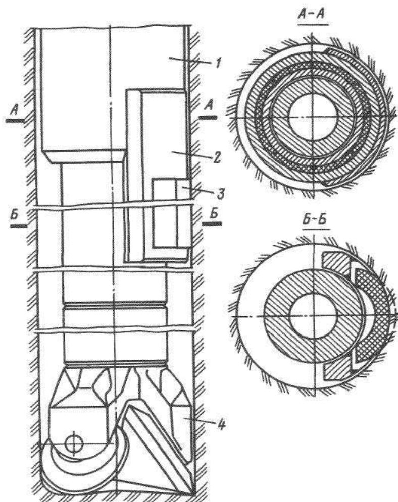
Рисунок 27 – Упругий отклонитель:
