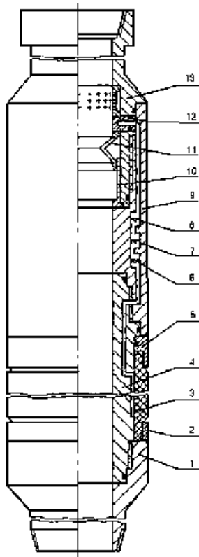
Рисунок 40- Пакер проходной гидравлический универсальный за колонный типа ППГУ:
