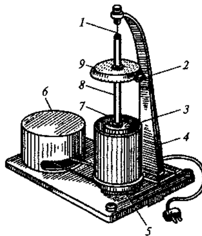
Рисунок 9 — Прибор СНС–2
