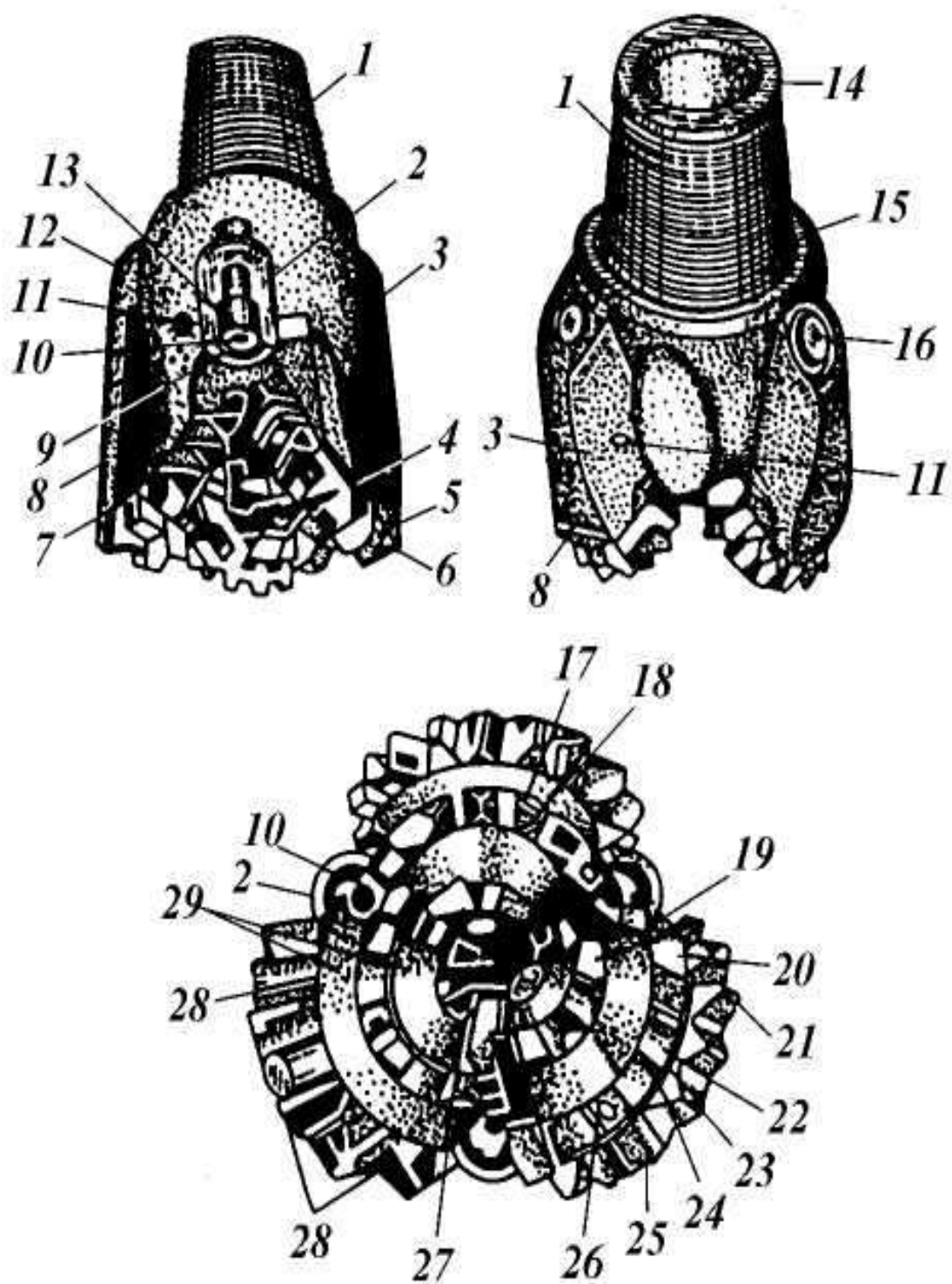
Рисунок 7 – Конструкция трехшарошечного долота
