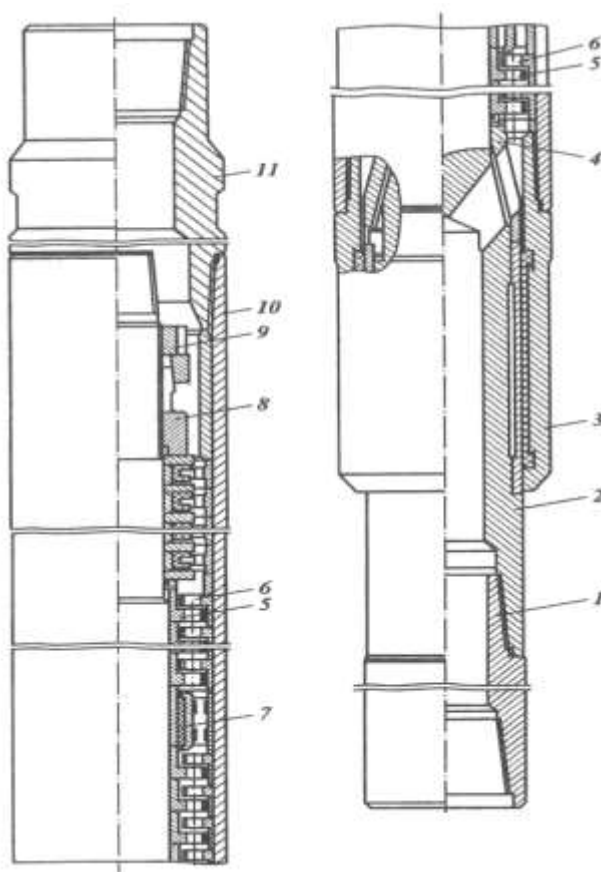
Рисунок 19 – Турбобур типа Т12МЗБ-240:
