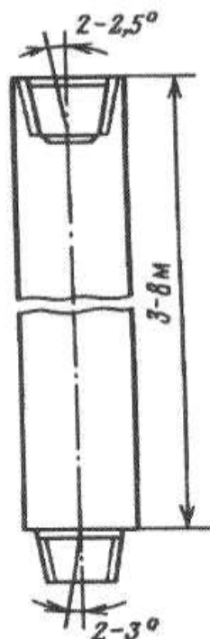
Рисунок 23 – Отклонитель Р-1
