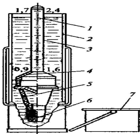
Рисунок 10 – Ареометр АГ–3ПП
