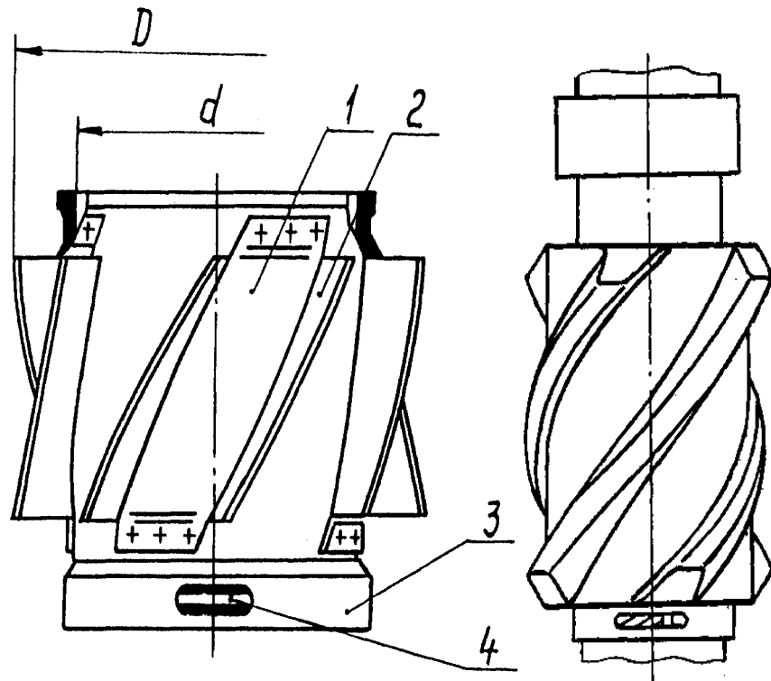
Рисунок 39 - Центраторы-турбулизаторы с упругими (ЦТ) и жесткими (ЦТГ) лопастями; 1-накладки; 2-упругие лопасти; 3-корпус; 4-винтовой клин.
