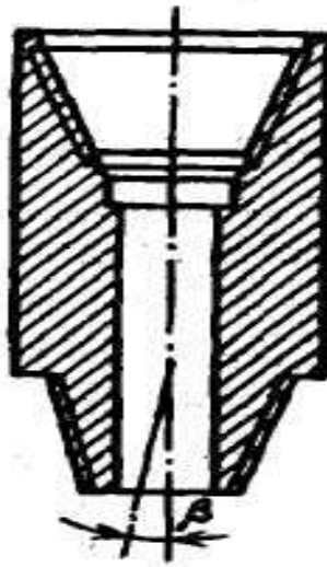
Рисунок 22 – Кривой переводник
