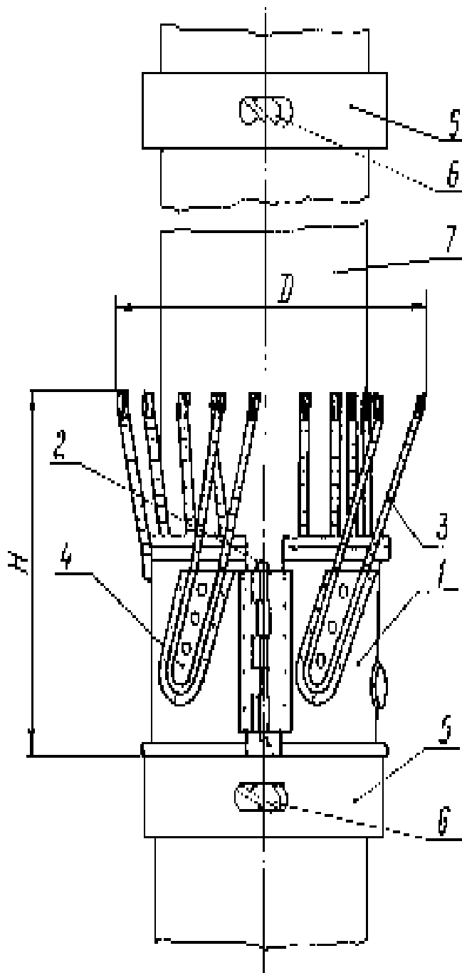
Рисунок 38 - Скребок корончатый типа СК:
