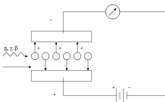
Рисунок 2.3 – Принципиальная схема работы ионизационной камеры
