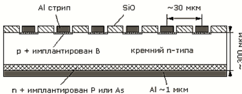
Рисунок 2.5 – Устройство кремниевого микроstriпового детектора
