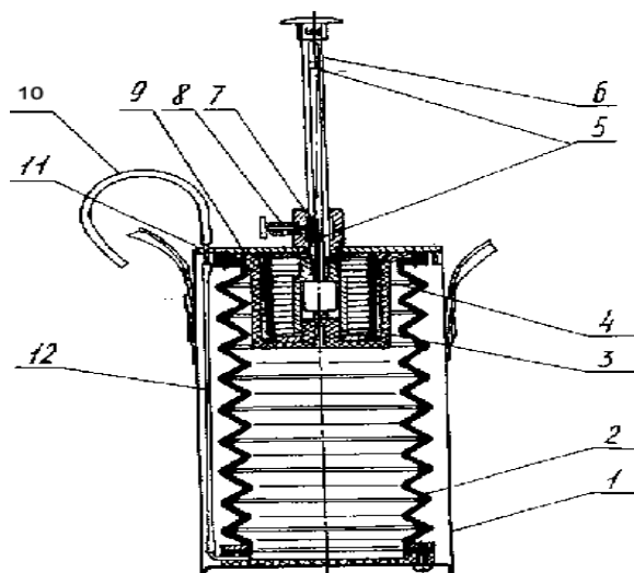
Рис. 12. Газоанализатор УГ-2
