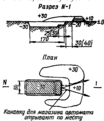
Одиночный окоп для стрельбы из автомата лежа
