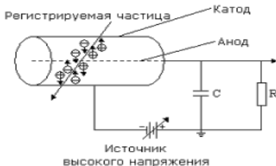
Рисунок 2. 4 – Принципиальная схема конструкции ГС
