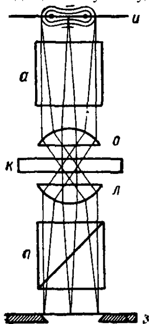
Рис. 34. Схема наблюдения интерференционной фигуры способом Лазо:
