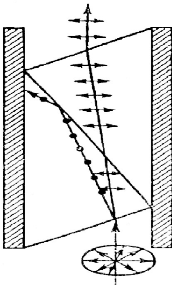
Рисунок 2. Ход лучей через призму Николя
