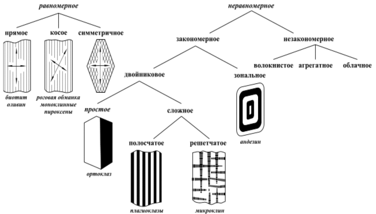
Рисунок 3.7 - Характер погасания минералов.
