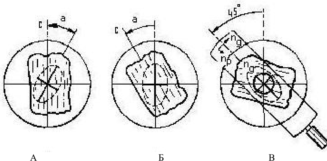
Рисунок 3.6 – Порядок определения угла погасания и наименования осей оптической индикатрисы минерала: А – спайность совмещена с вертикальной нитью окулярного креста; Б – минерал на погасании; В – определение наименования оси индикатрисы
