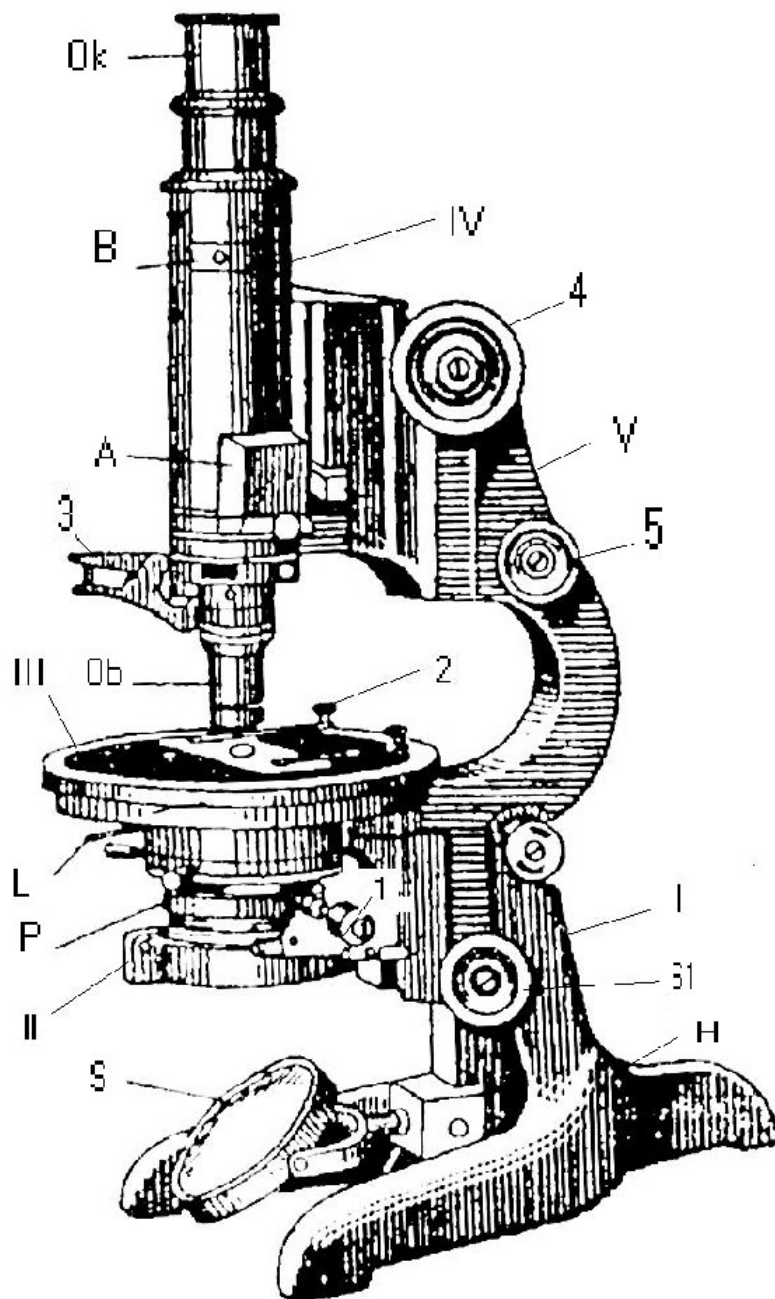
Рисунок 1. Поляризационный микроскоп МП-3
