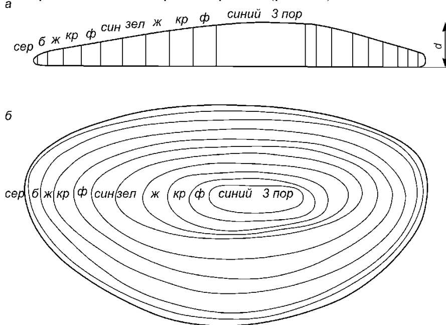
Рисунок –3.2 Зависимость между толщиной зерна ( d ), разностью хода ( R ) и интерференционной окраской a – поперечный разрез; b – вид сверху.
