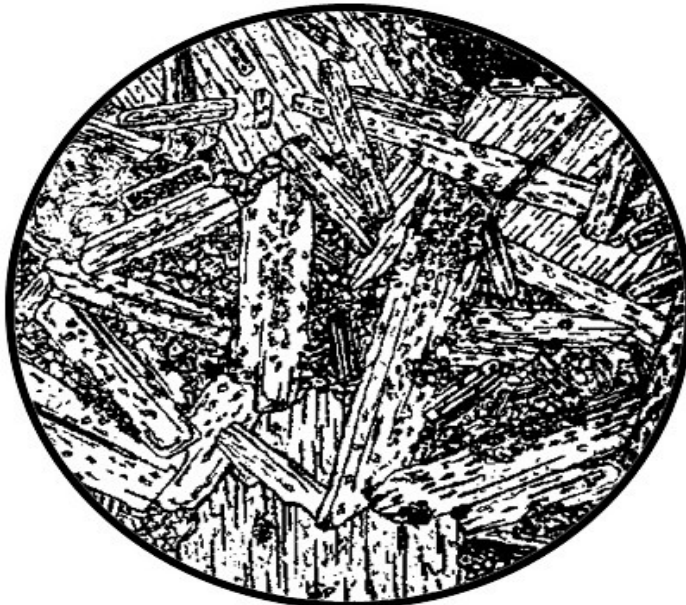
Рисунок 14.2 - Диабаз
