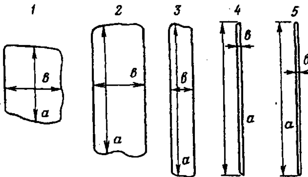
Рисунок 5. Форма зерен кристаллов: 1 - изометрическая, a/b=1 ; 2 - таблитчатая, a/b от 2 до 4; 3 - призматическая, a/b - от 4 до 10; 4 - шестовая, a/b от 10 до 20; 5 - игольчатая, a/b > 20 .
