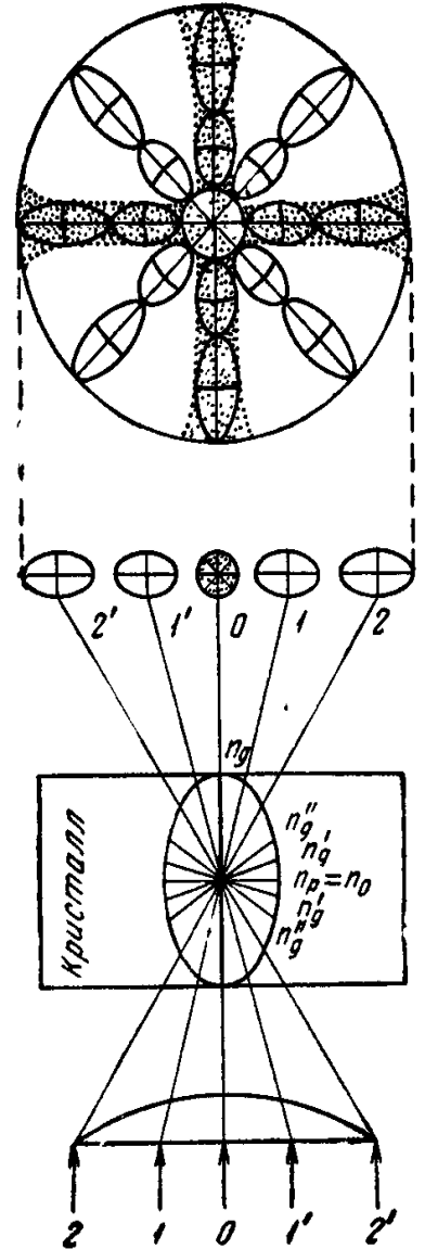
Рис. 35. Схема получения интерференционной фигуры одноосного оптически положительного минерала на разрезе, перпендикулярном к оптической оси.
