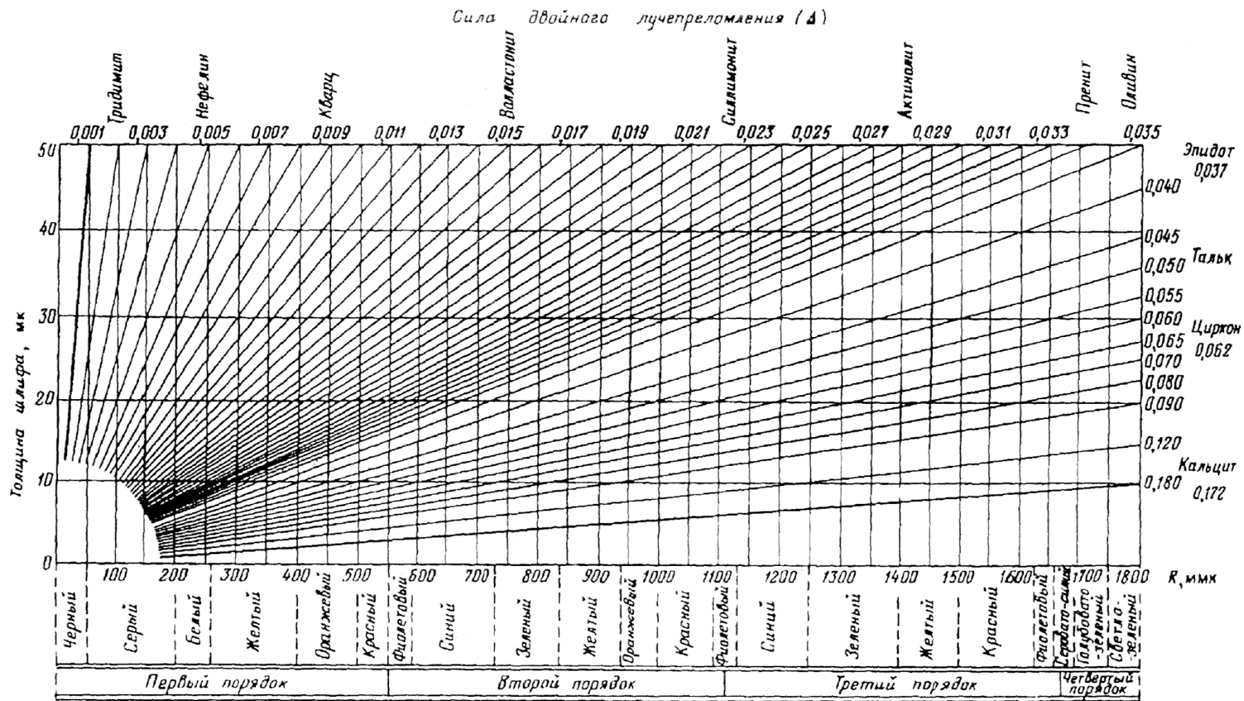
Рисунок 3.1 - Номограмма Мишель-Леви
