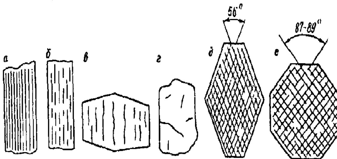
Рисунок 6. Типы спайности
