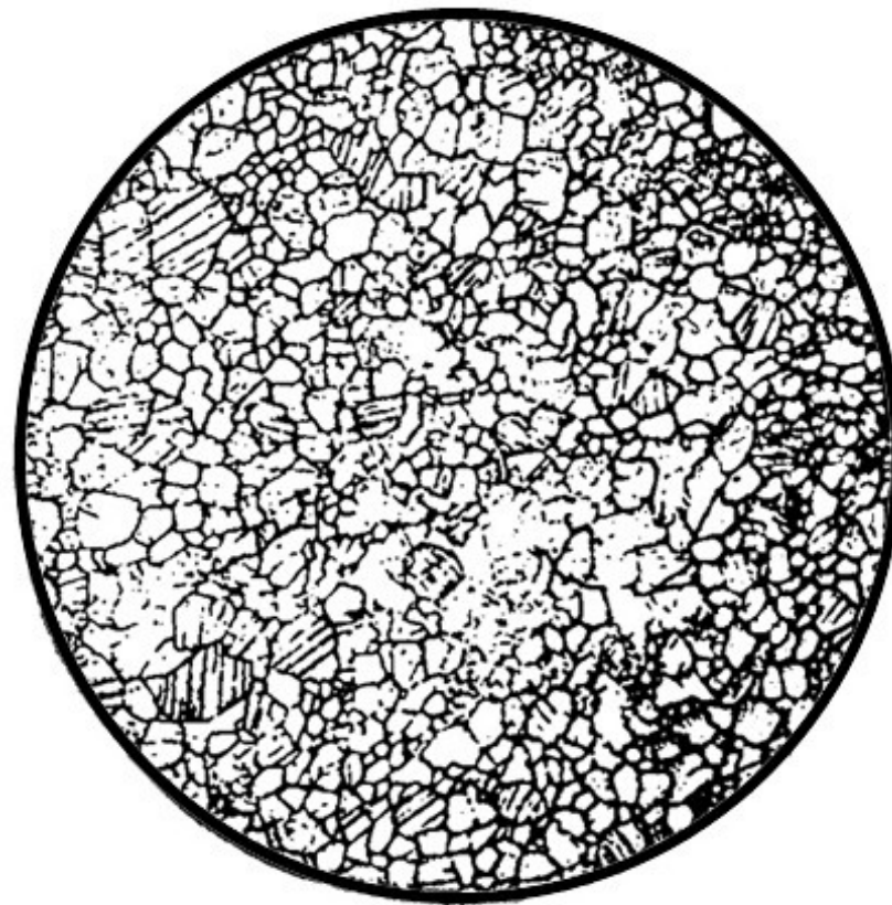
Рисунок 16.2 - Гомеобластовая структура
