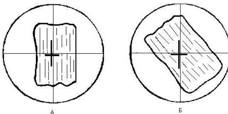
Рисунок 3.5 – Характер погасания
