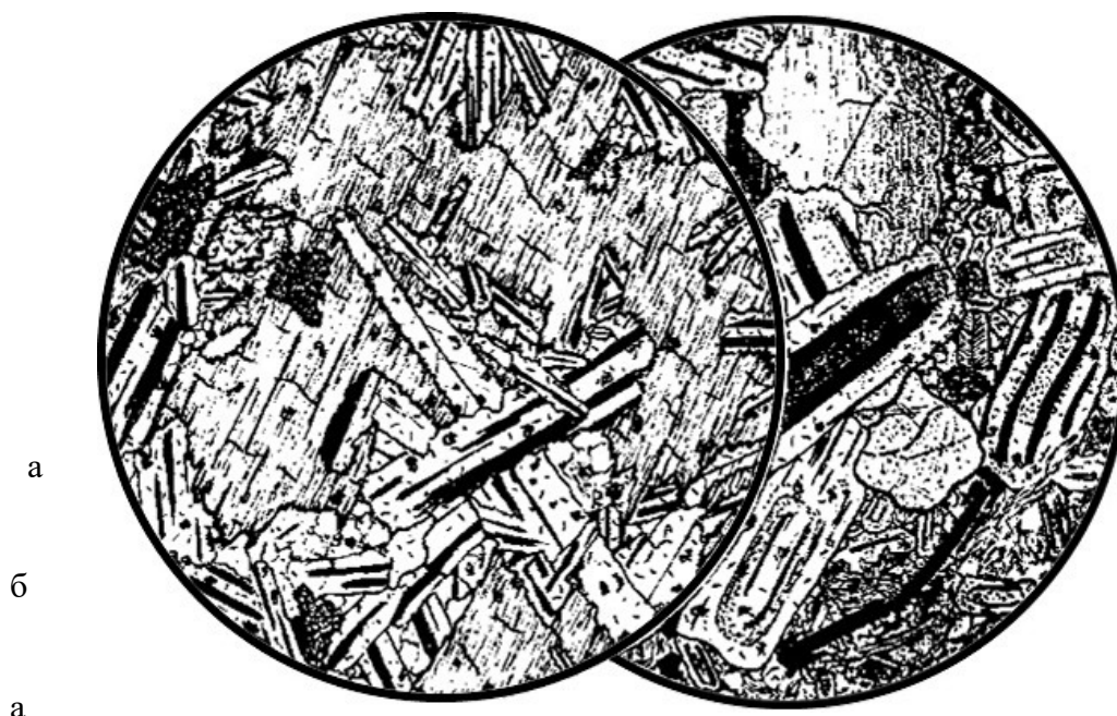
Рисунок 14.1 - -диабаз; б –
