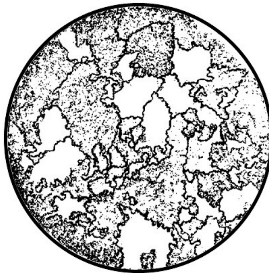
Рисунок 16.7 – Зубчатая структура
