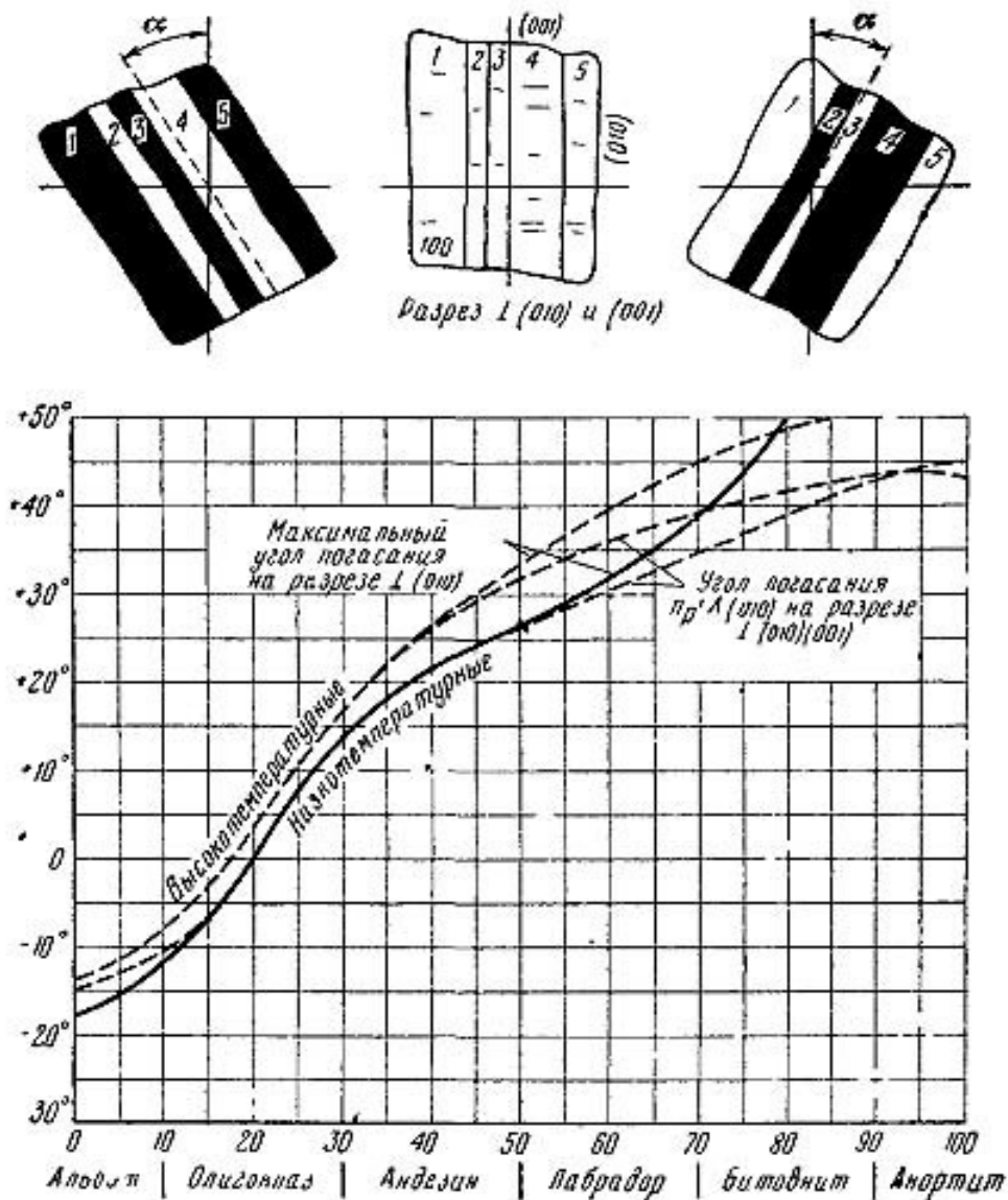
Рисунок 5.1 – Диаграмма для определения состава плагиоклазов
