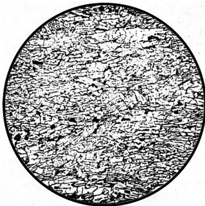
Рисунок 16.5 – Нематобластовая структура
