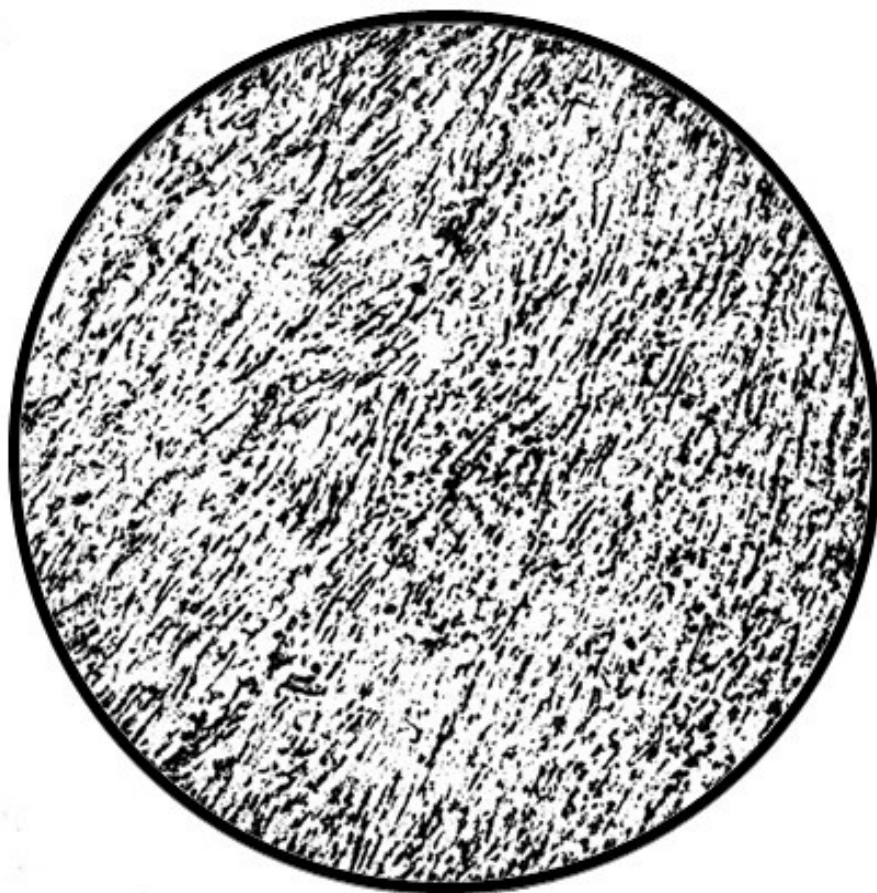
Рисунок 16.6 – Фибробластовая структура
