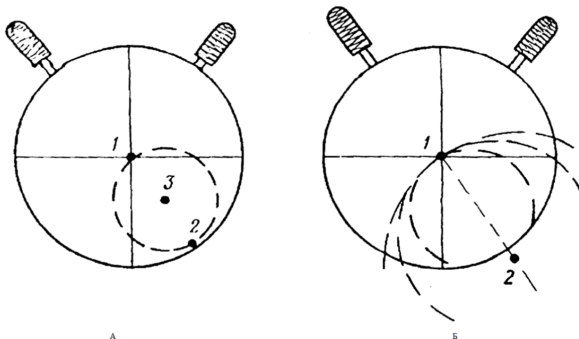
Рисунок 3. Схема центрировки микроскопа
