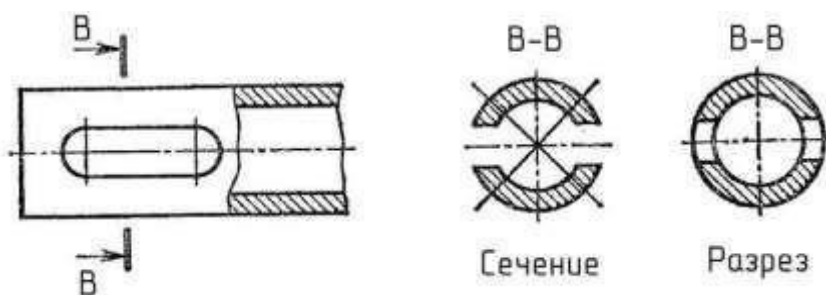
Рисунок 24.4 – Сечение не круглого отверстия
