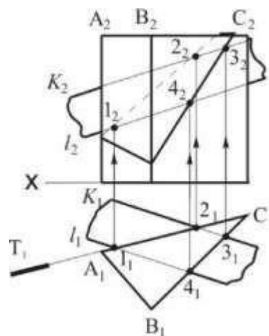
Рисунок 7.2 — Прямая призма (способ граней)
