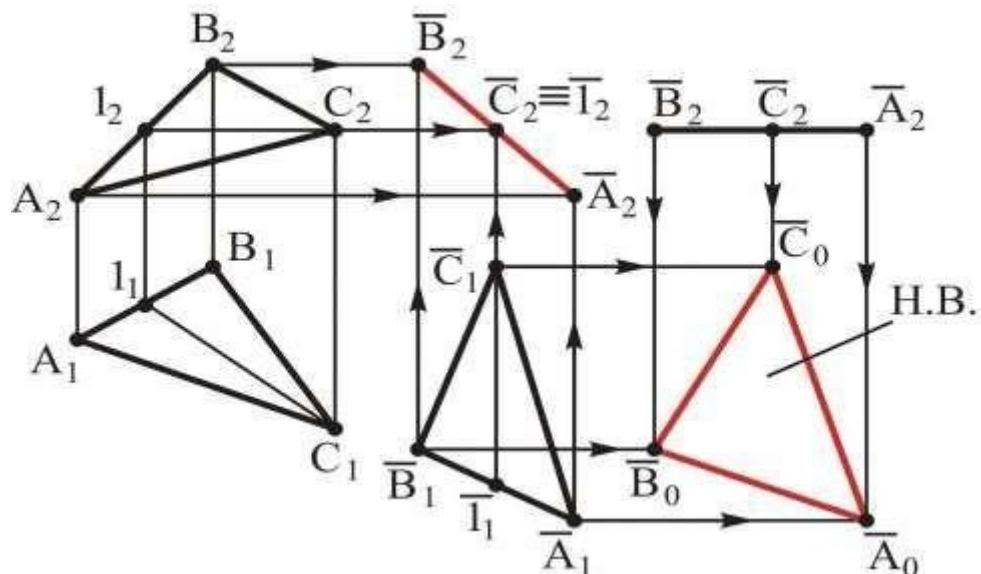
Рисунок 6.6 – Перемещение фигуры
