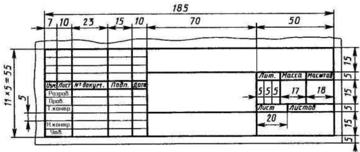
Рисунок 10.2 – Основная надпись
