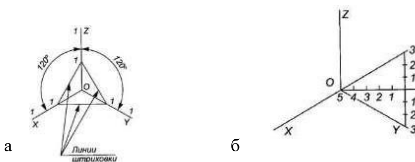
Рисунок 20.6 – Оси координат в изометрии
