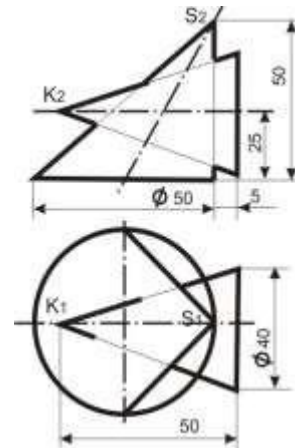
Рисунок— Два конуса
