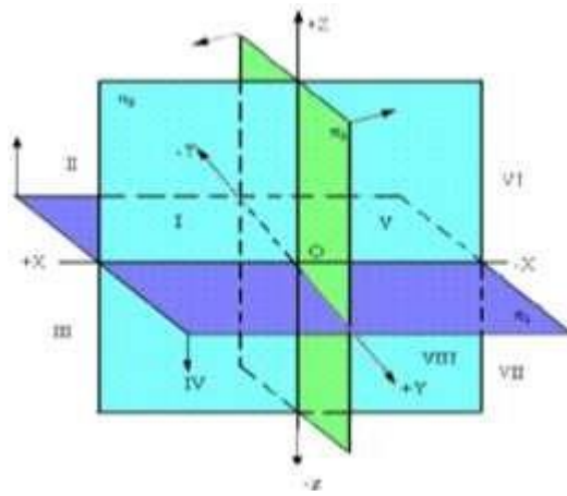
Рисунок 1.1 – Октанты пространства
