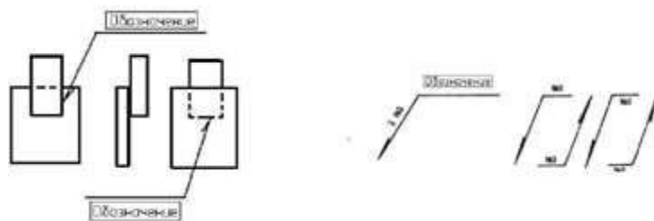
Рисунок 27.3 – Обозначение швов
