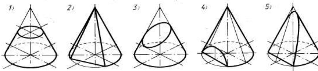
Рисунок 8.1. — Сечения конуса
