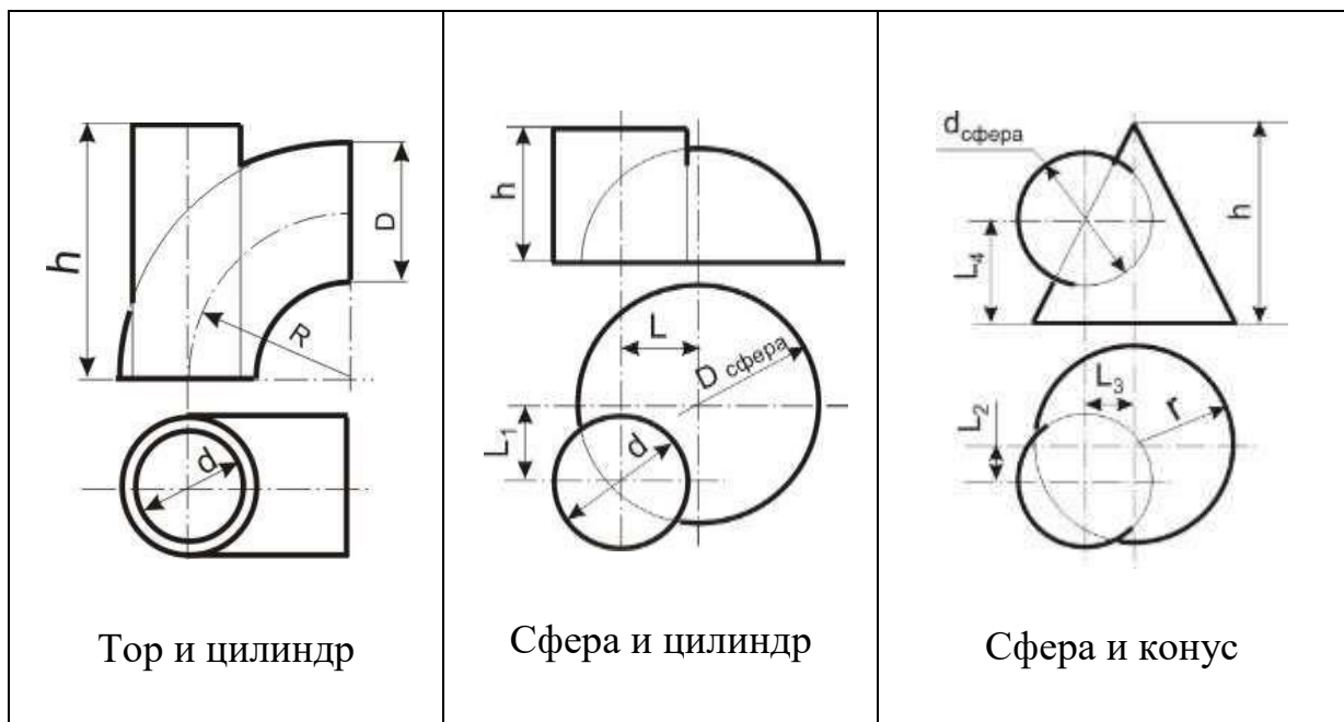
Рисунок 9.3 — Пересечение поверхностей вращения
