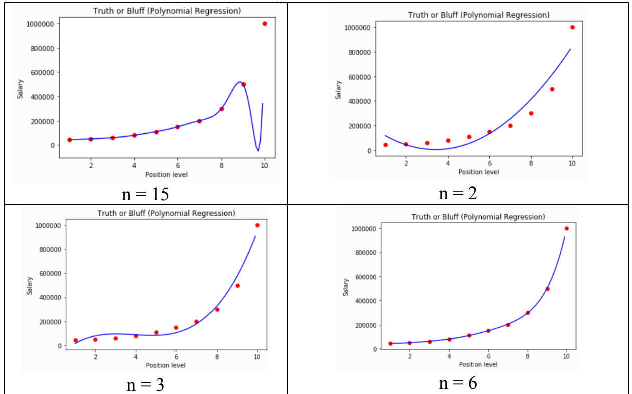
Рисунок 8.2 – Анализ модели полиномиальной регрессии
