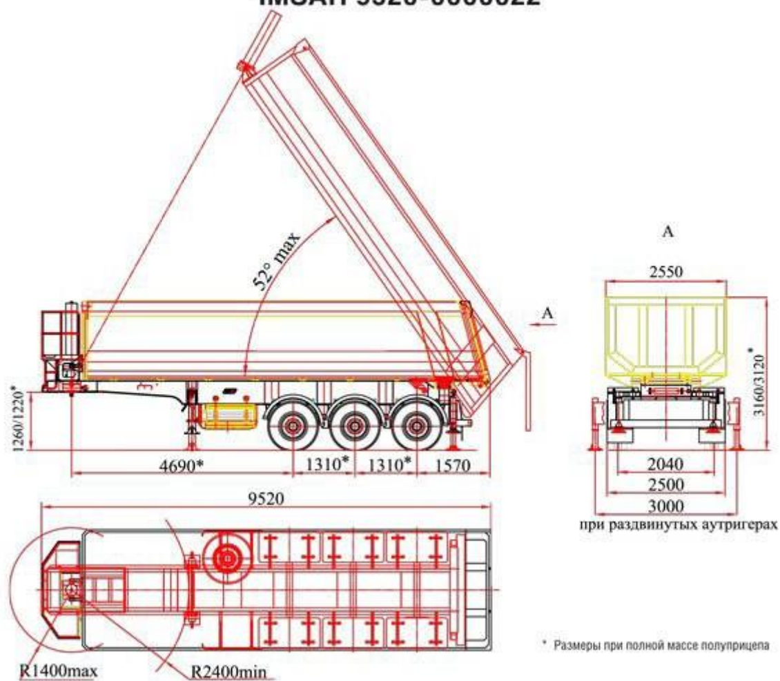
Рисунок 3В - Самосвальный полуприцеп ЧМЗАП 9520-022
