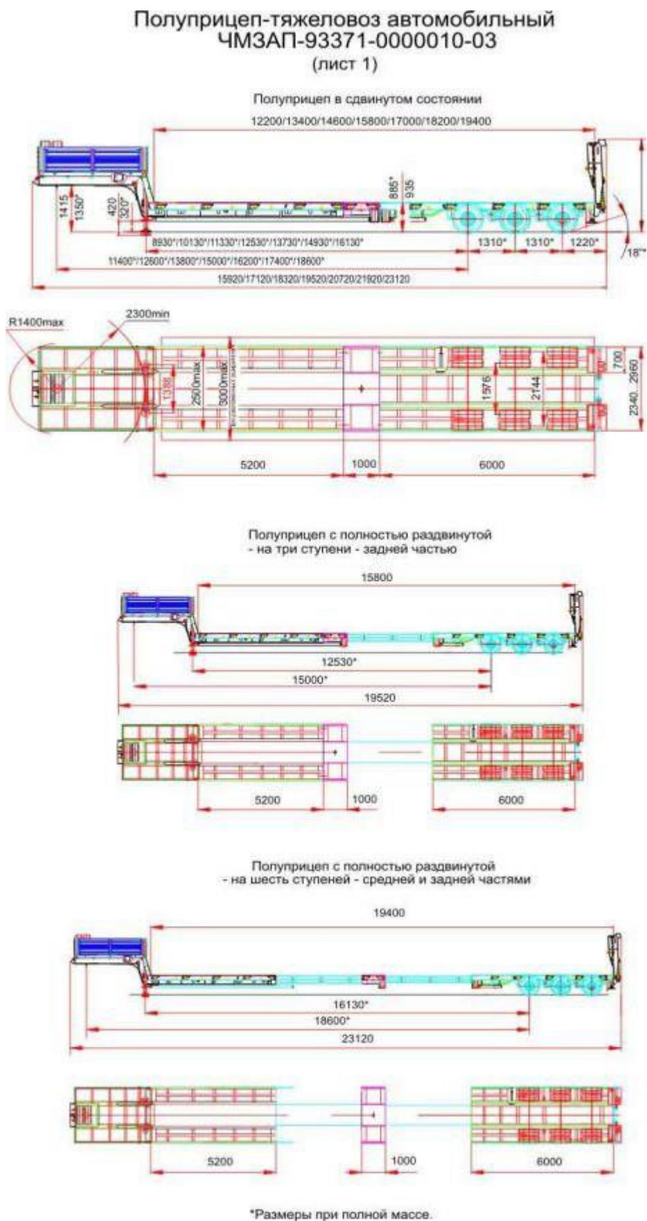
Рисунок 2Г - Полуприцеп – тяжеловоз ЧМЗАП 93371-010-03
