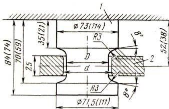
Рисунок 1 - Номинальные размеры сцепного шкворня 1 и захватов 2 (Размеры без скобок даны для полуприцепов полной массой до 40т, а в скобках для полуприцепов полной массой более 40т)
