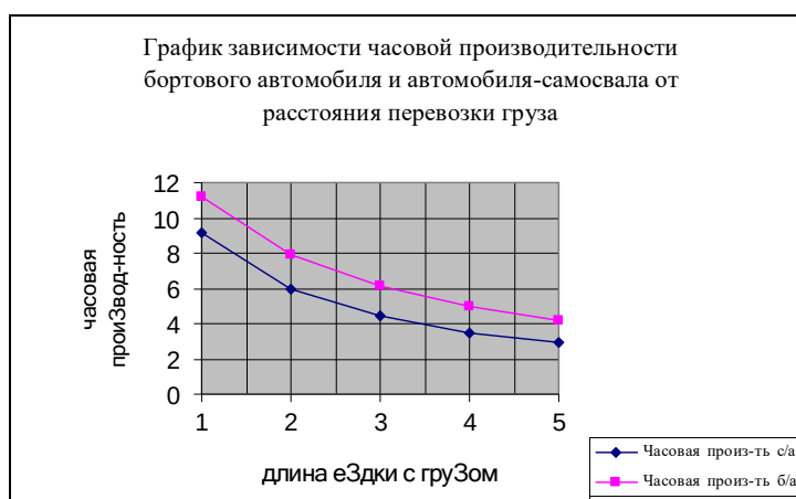
Рис. 2.1. Пример построения графика часовой производительности автомобилей
