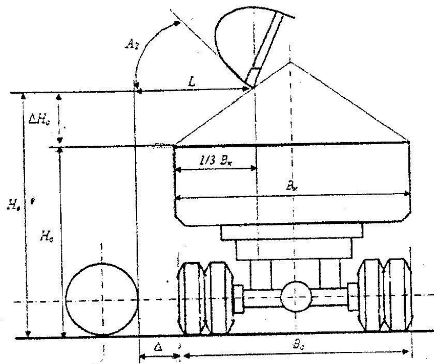
Рисунок 5 - Схема загрузки кузова самосвала погрузчиком
