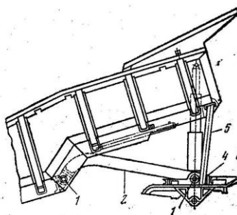
Рисунок 8 – Полуприцеп - самосвал
