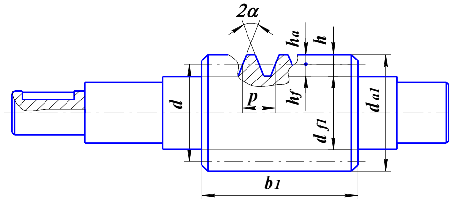
Рис. 4.1 – Червяк
