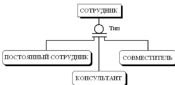
Рисунок 4.6 - Пример полной категории
