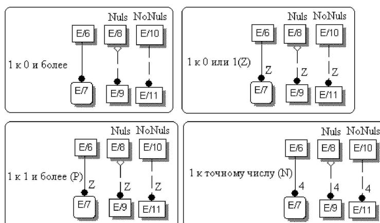
Рисунок 4.18 - Изображение связей в нотации IDEF1X. Помимо типа связи, на диаграмме могут отображаться и установки ссылочной целостности - для этого необходимо выбрать в контекстном меню диаграммы пункт Relationship Display и подпункт Referential Integrity (рисунок 4.19).
