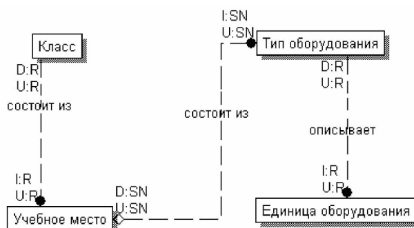
Рисунок 4.20 - ER-диаграмма с включенными установками ссылочной целостности. На диаграмме теперь определена одна из объектных областей, которых
