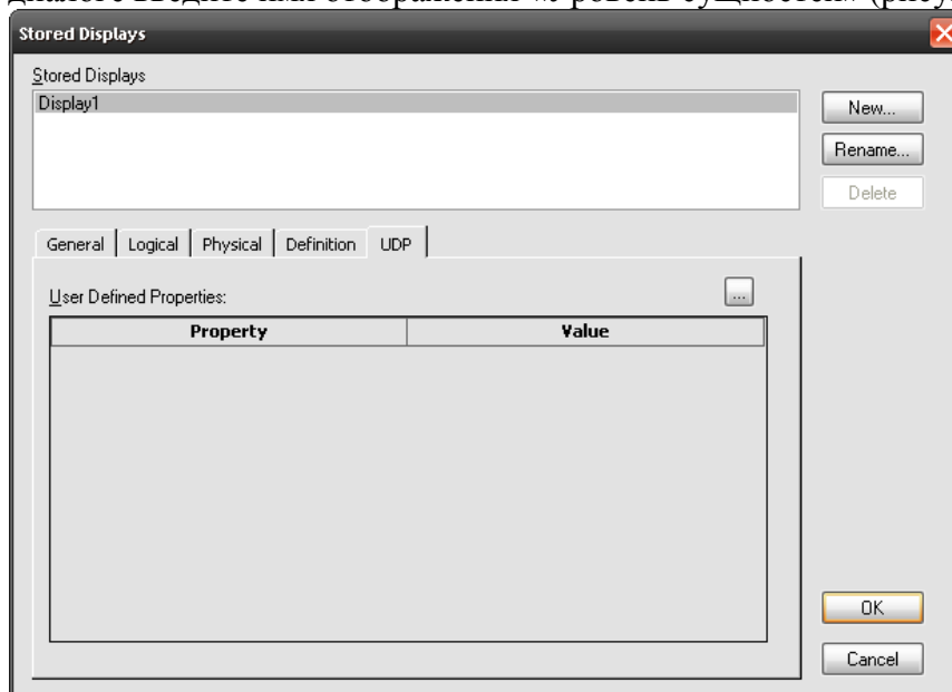
Рисунок 2.29 - Закладка UDP
