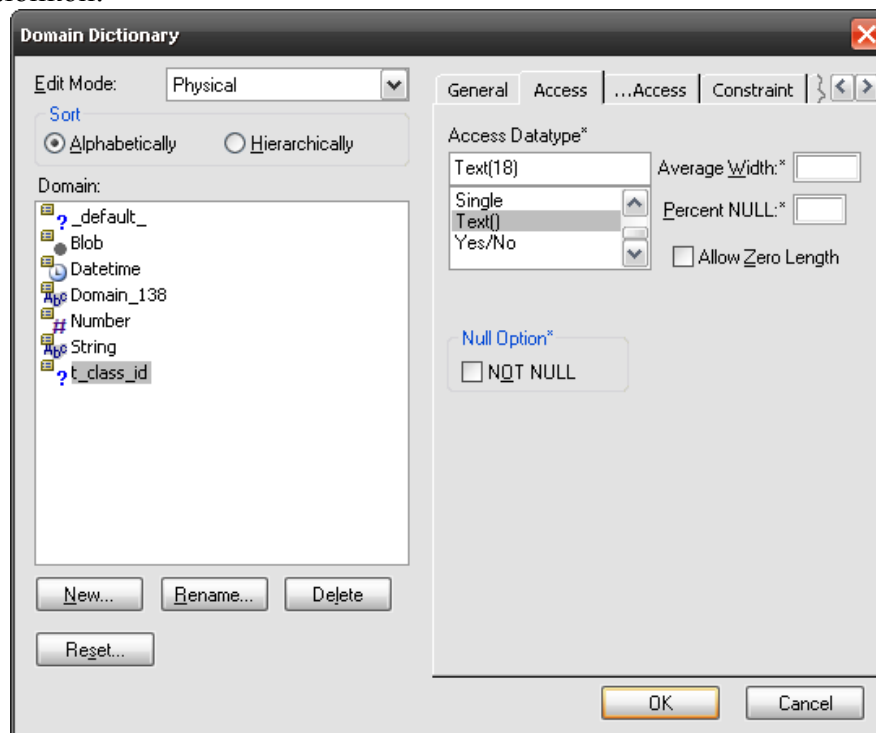
Рисунок 3.15 - Страница Access
