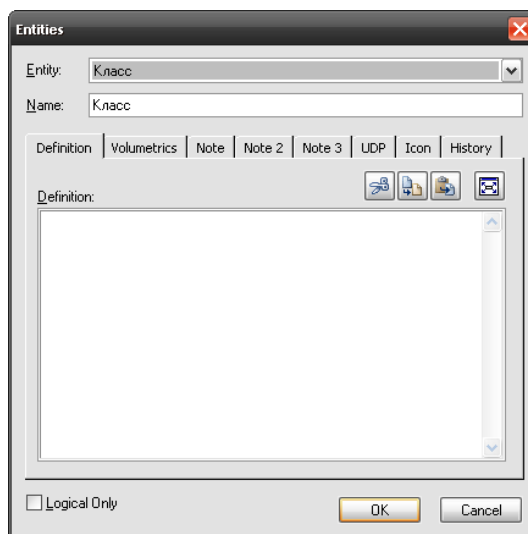
Рисунок 3.5 –Редактор сущности
