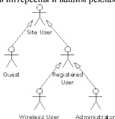
Рис. 1: Иерархия исполнитель-роль
