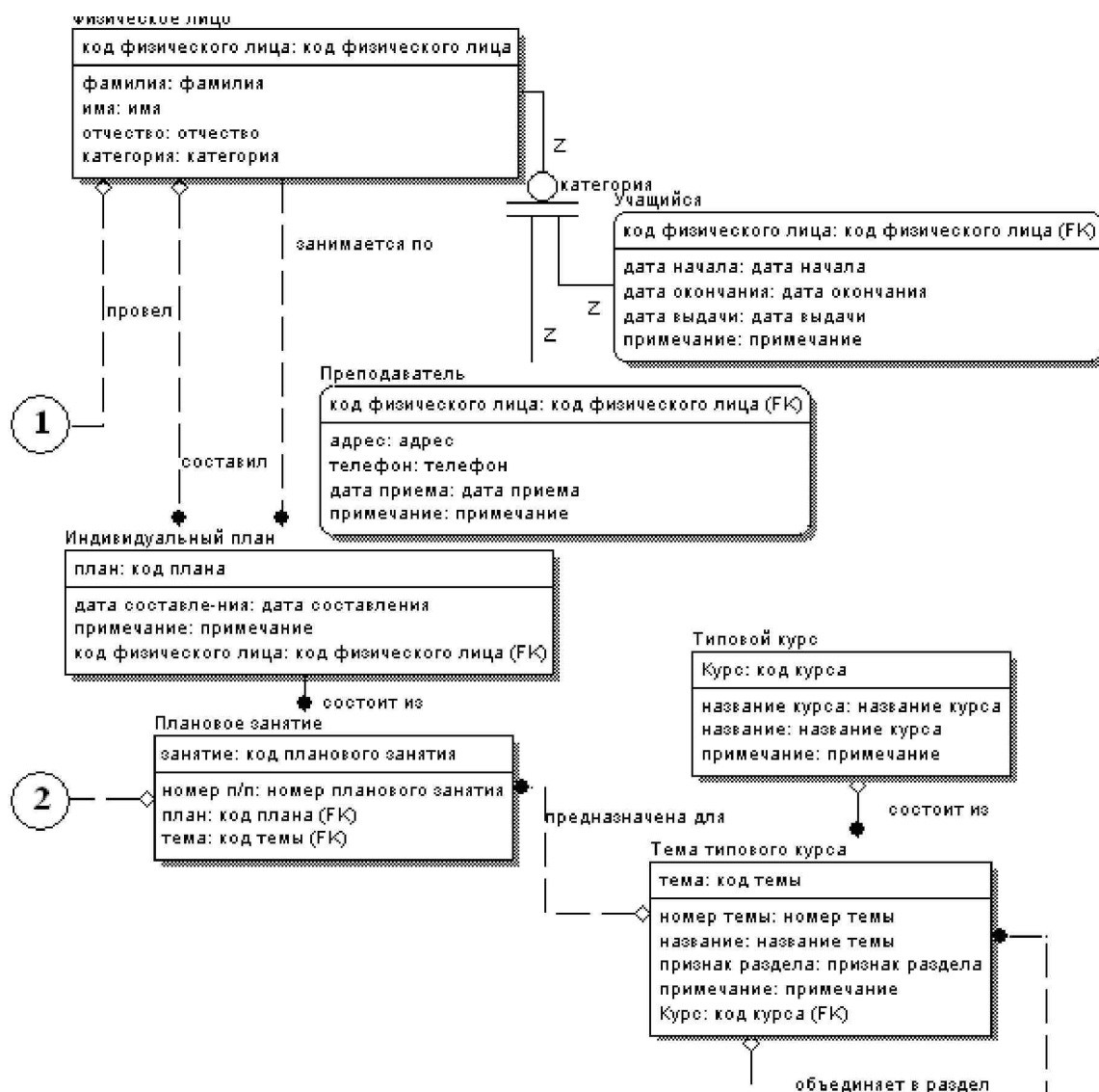
Рисунок 5.12 –ER-диаграмма после введения сущности «Занятие в классе». Уровень
