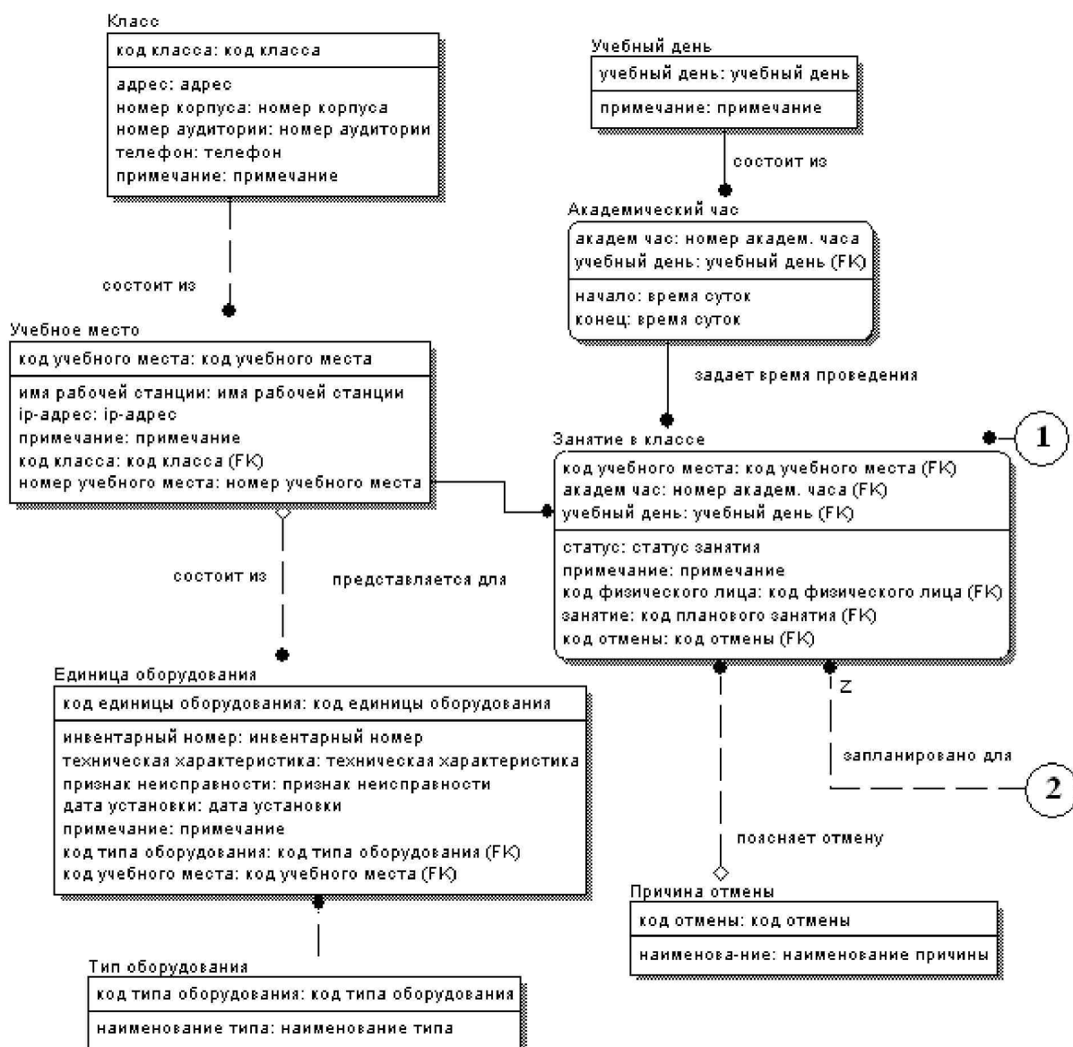
Рисунок 5.11 – ER-диаграмма после введения сущности «Занятие в классе». Уровень атрибутов (лист 1)
