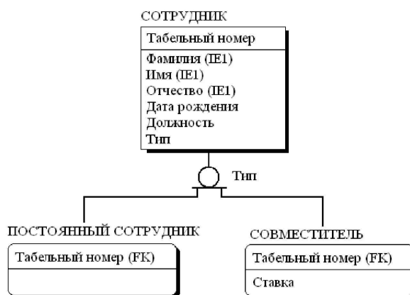
Рисунок 4.5 - Пример неполной категории
