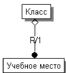
Рисунок 4.8 - Неидентифицирующая связь
