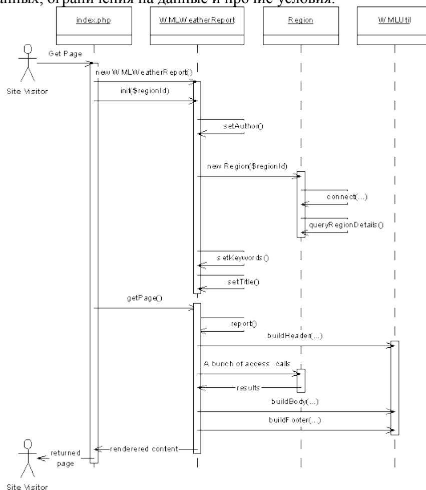
Рис. 7. Диаграмма последовательностей
