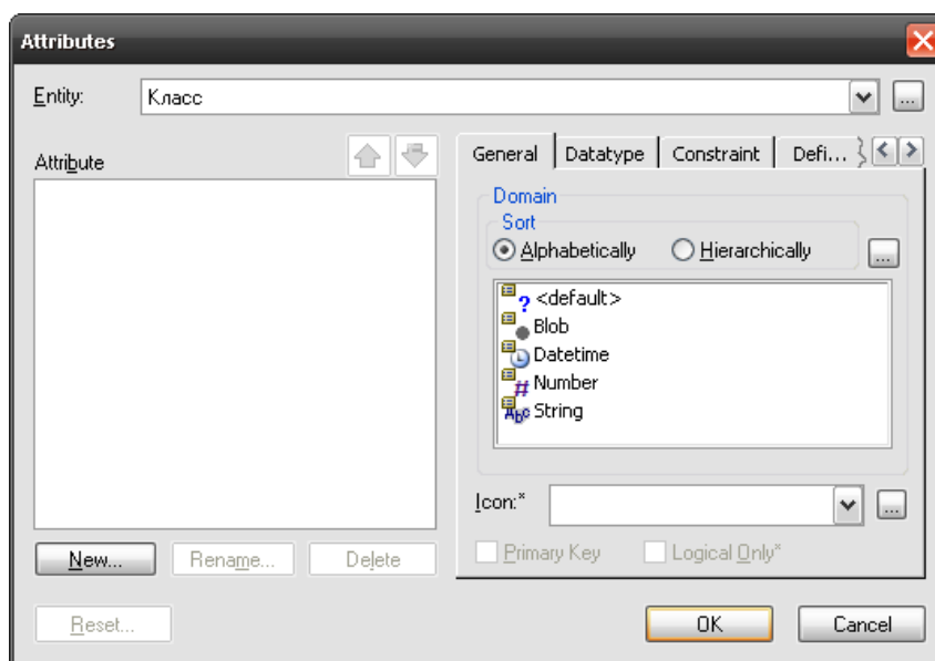
Рисунок 3.16 – Редактор атрибутов
