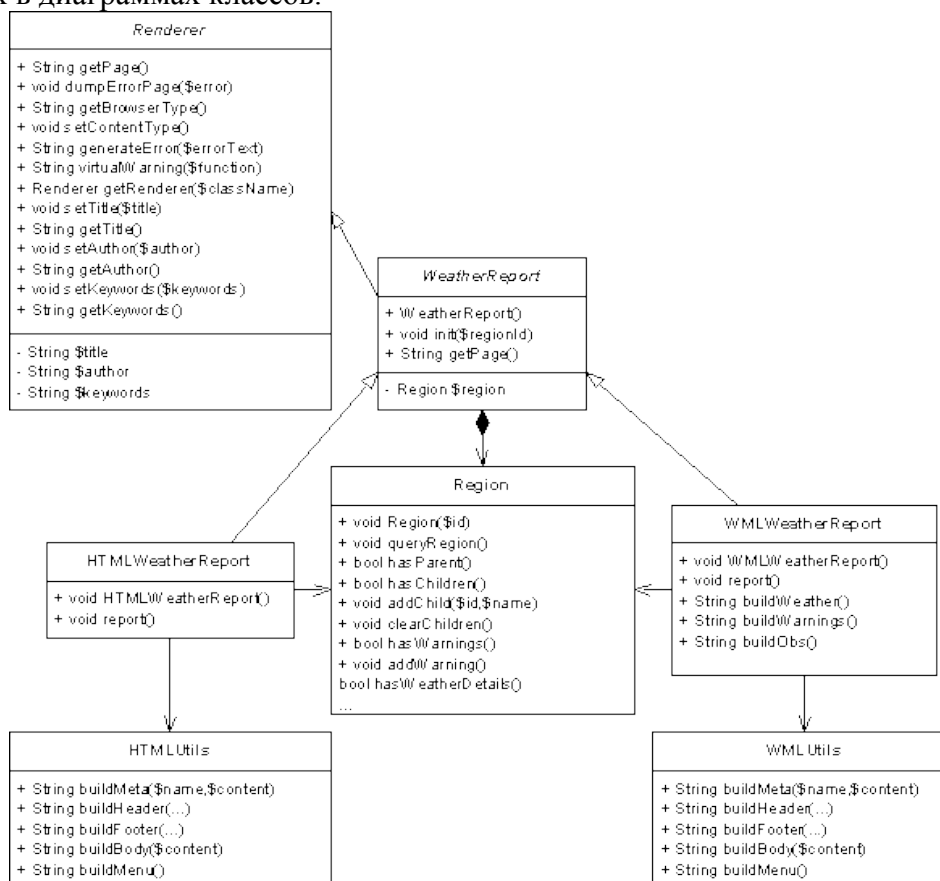
Рис. 5: Диаграмма классов
