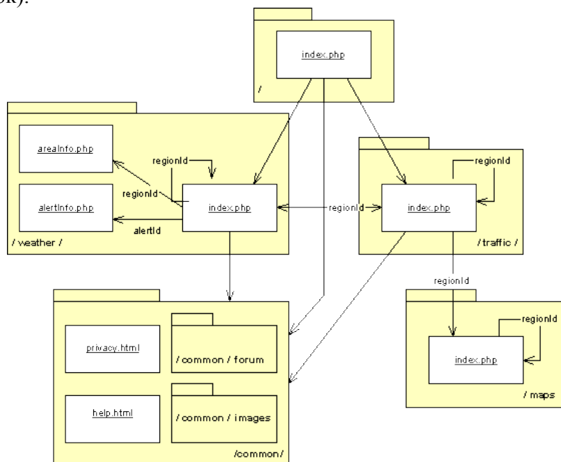
Рис. 3: Диаграмма страниц
