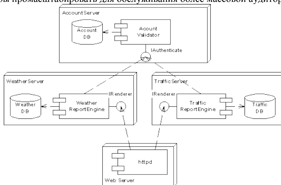
Рис.8: Диаграмма компонентов
