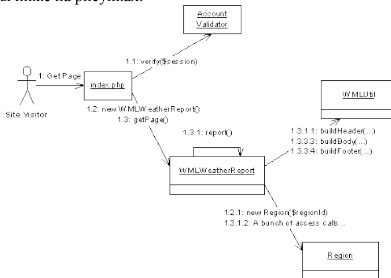
Рис. 6. Диаграмма взаимодействия.
