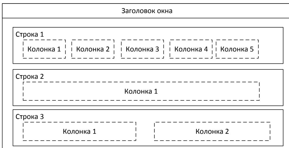
Рисунок 6.2 – Сетка размещения элементов управления в PySimpleGUI
