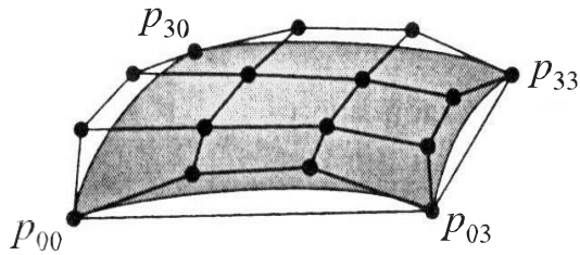
Рис. 5.5 – Порция поверхности Безье
