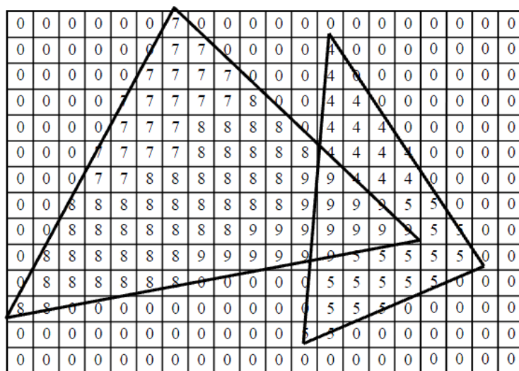
Рис. 4.12 – Организация Z-буфера
