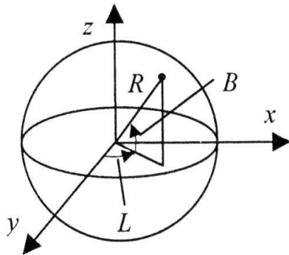
Рис. 4.21 – Широта и долгота
