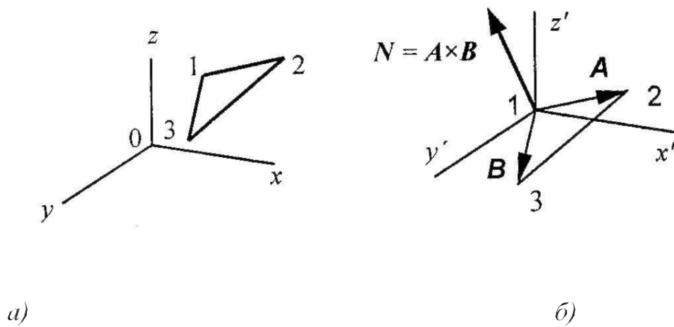
Рис. 4.17 – Пример плоской грани поверхности: а — треугольная грань, б — радиус-векторы
