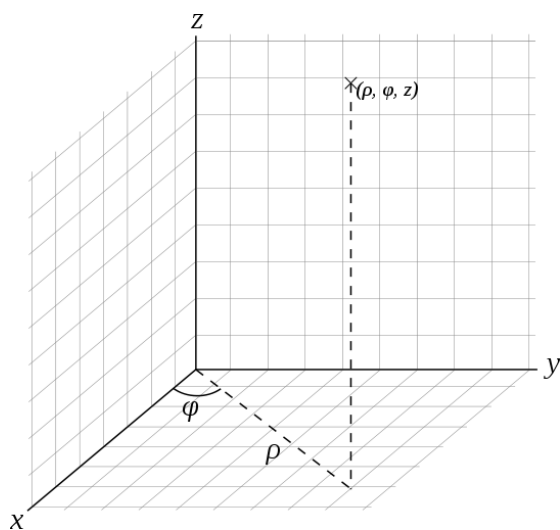
Рис. 2.7 – Цилиндрическая система координат
