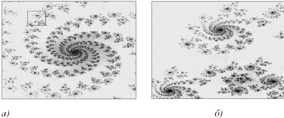
Рис. 1.6 – Пример фрактального изображения
