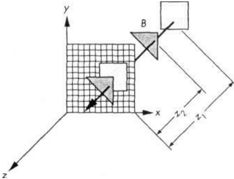
Рис. 4.13 – Алгоритм Z-буфера
