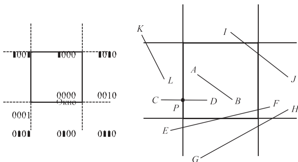
Рис. 3.2 – Окно отсечения и прилегающие к нему части плоскости
