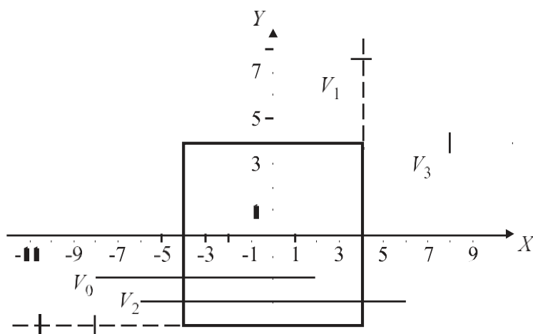
Рис. 3.3 – Пример расчета отсечения в алгоритме Лианга—Барского
