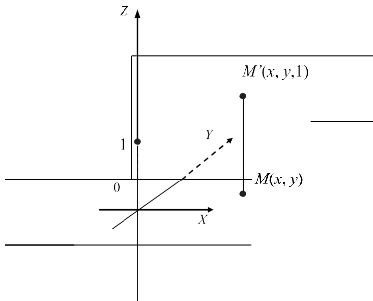
Рис. 2.11 – Однородные координаты
