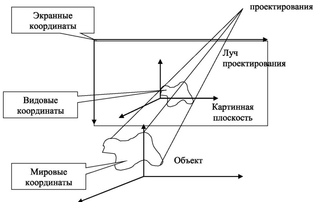
Рис. 4.2 – Проектирование
