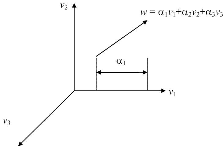
Рис. 2.5 – Представление вектора
