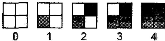
Рис. 3.15 – Ячейки 2 \times 2
