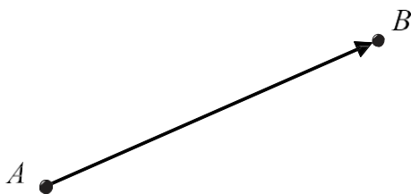
Рис. 2.1 – Соединение двух точек вектором
