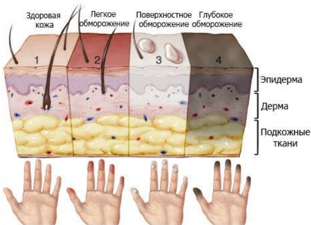
Рисунок 6.1. Степени отморожения
