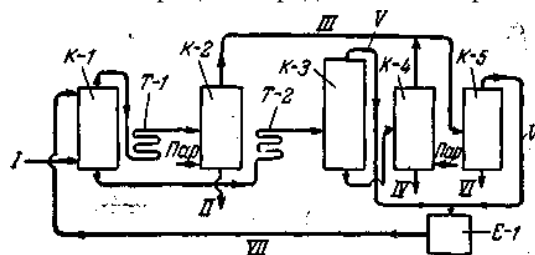
Рисунок 1 – Принципиальная схема очистки масел избирательными растворителями:
