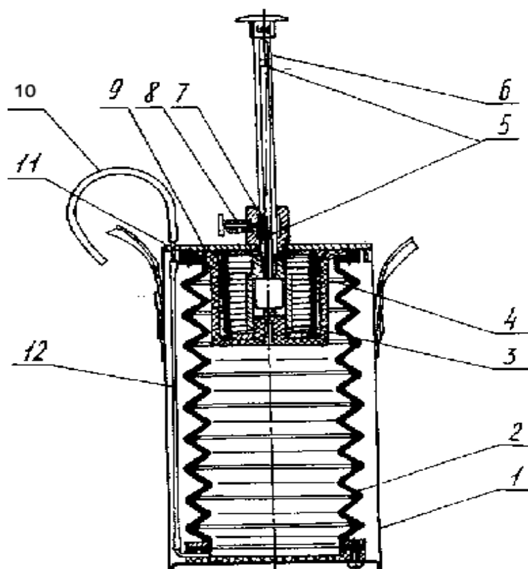
Рисунок 3.1– Устройство газоанализатора УГ-2: 1 – корпус. 2 – сильфон, 3 – пружина, - кольцо распорное, 5 – канавка с двумя углублениями, 6 – шток, 7 – втулка, 8 – фиксатор, 9 – плата, 10 – трубка резиновая, 11 – штуцер, 12 – трубка резиновая
