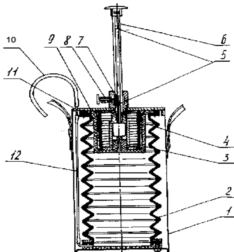
Рисунок 3 .1– Устройство газоанализатора УГ-2: 1 – корпус. 2 – сильфон, 3 – пружина, - кольцо распорное, 5 – канавка с двумя углублениями, 6 – шток, 7 – втулка, 8 – фиксатор, 9 – плата, 10 – трубка резиновая, 11 – штуцер, 12 – трубка резиновая
