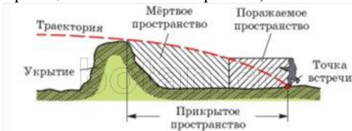
Рис. 52. Прикрытое, поражаемое и мёртвое пространство
