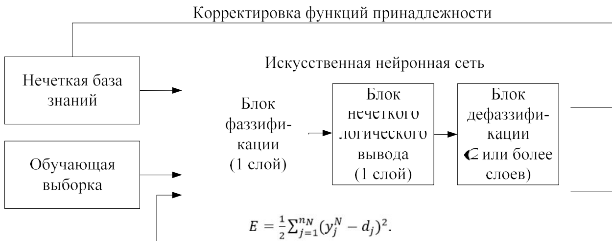
Рис. 4.1. Общая структура гибридной нейро-нечеткой системы Система
