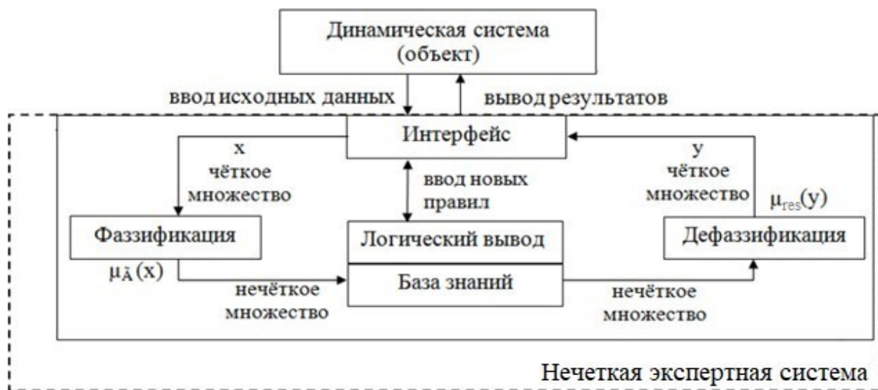
Рис. 1.2. Структура НЭС
