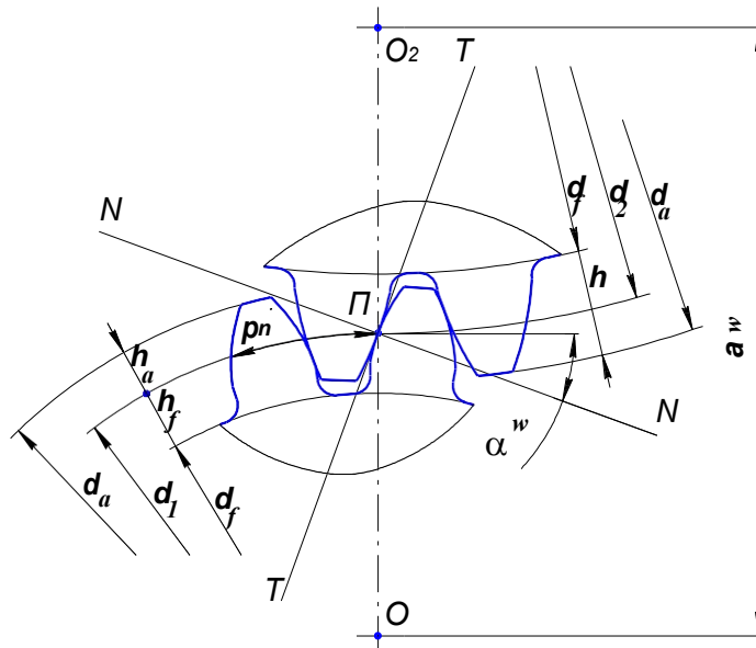
Рис. 3.1 – Зубчатое зацепление
