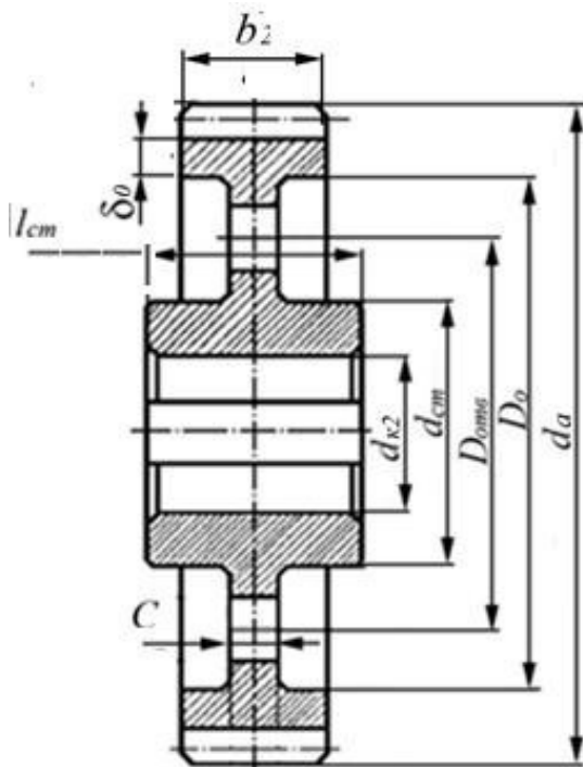
Рисунок 6 – Схема колеса
