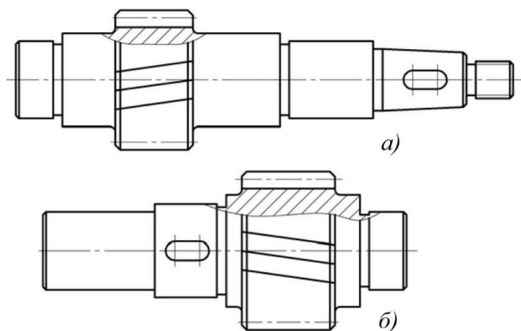
Рисунок 2 – Конструкции вал-шестерни
