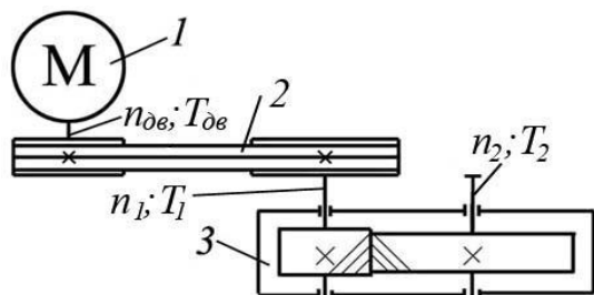
Рисунок 7 – Приводная станция: 1 – электродвигатель; 2 – клиноременная передача; 3 – редуктор
