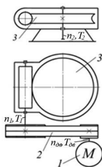
Рисунок 1 – Приводная станция:
