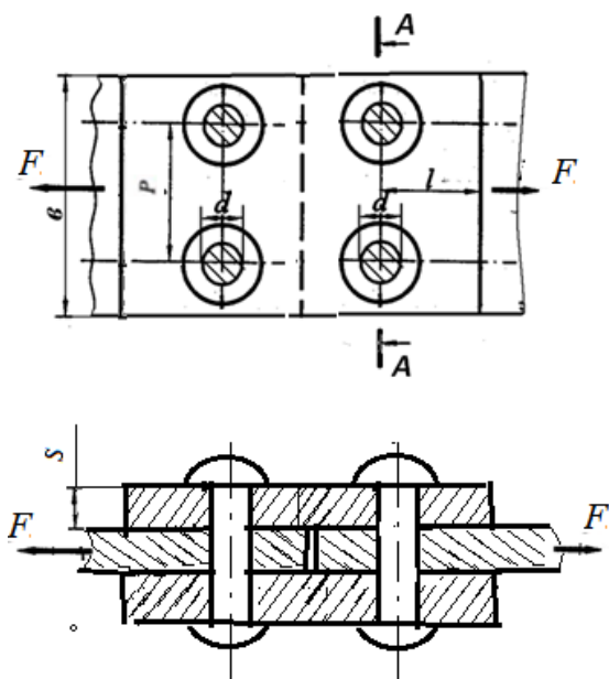
Рисунок 2-Заклепочный шов
