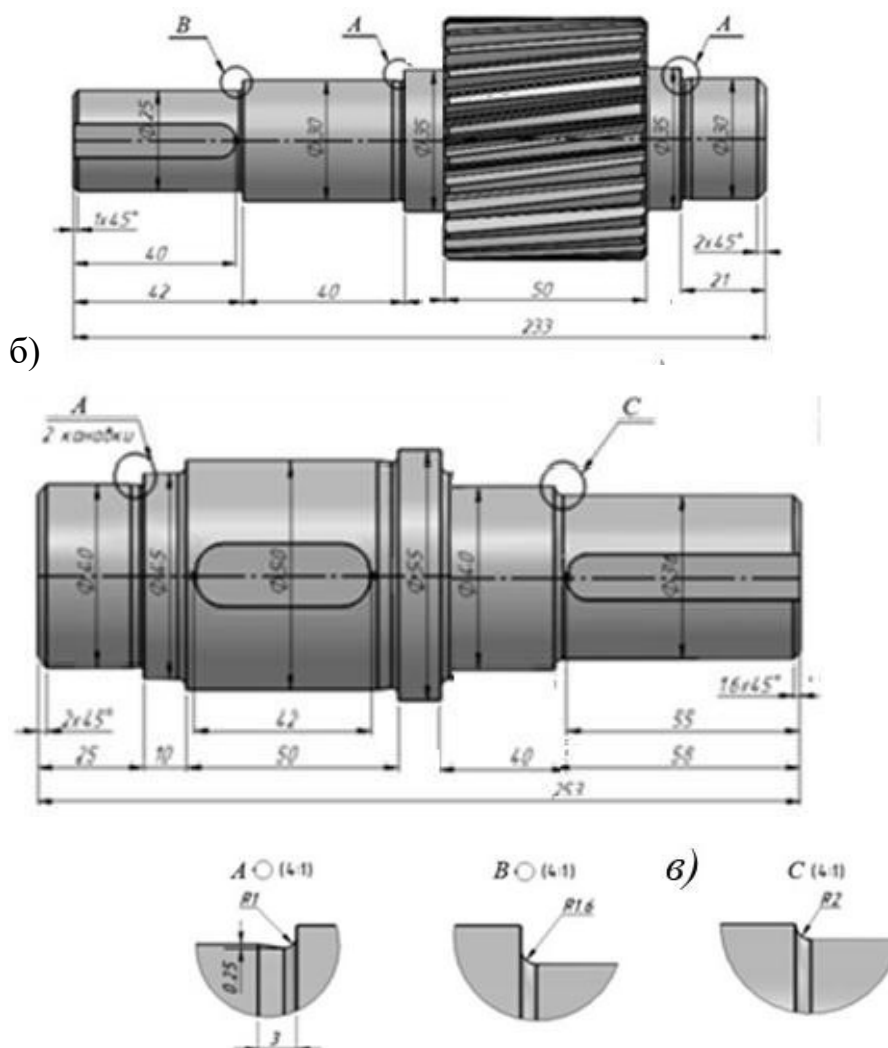
Рисунок 3 – Примеры конструктивного исполнение валов: а – ведущий вал в сборе с подшипниками; б – ведущий вал; в – ведомый вал
