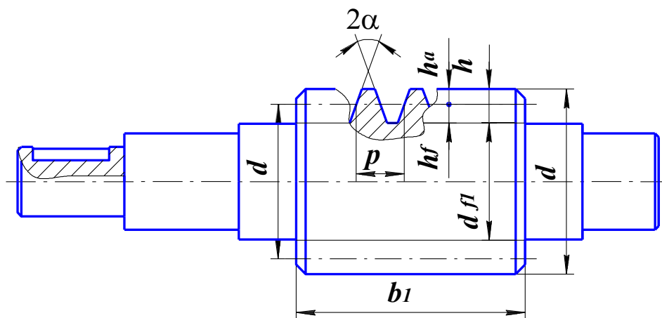
Рис. 3.1 – Червяк
