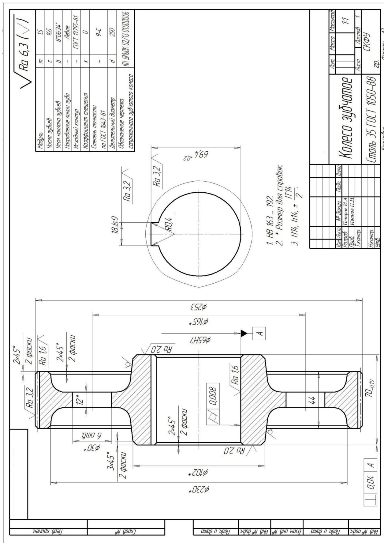
Рисунок 4 – Рабочий чертеж цилиндрического колеса
