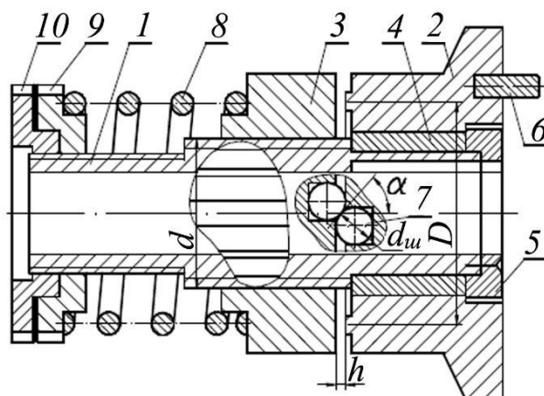
Рисунок 9.2 – Пружинно-шариковая муфта
