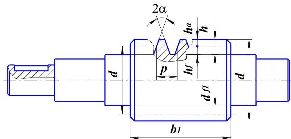
Рис. 4.1 – Червяк
