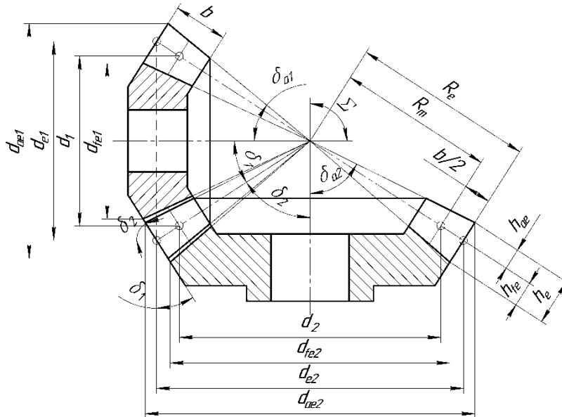
Рисунок 3 –Схема конического зацепления Делительные диаметры зубчатых колес
