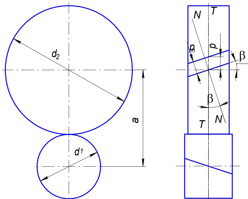
Рис. 3.2 – Косозубая передача
