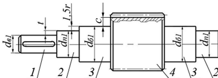
Рисунок 1 – Схема ведущего вала
