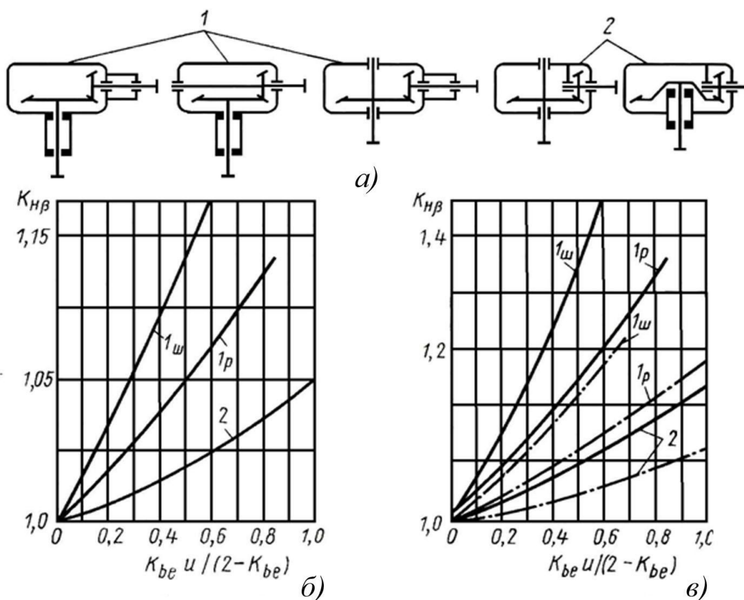
Рисунок 1 – Графики для определения коэффициента K_{H\beta} конических передач с прямыми зубьями (сплошные линии) и круговыми зубьями (штрих пунктирные линии) при коэффициенте K_{be} = 0,285
