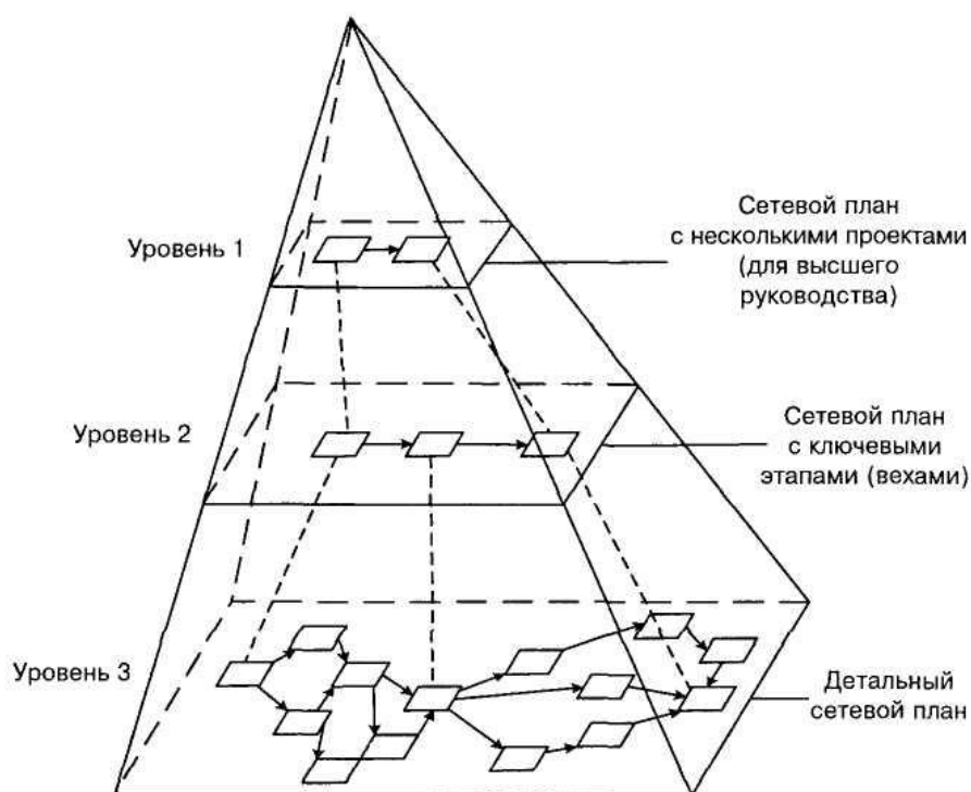
Рисунок 3.1 – Уровни планирования
