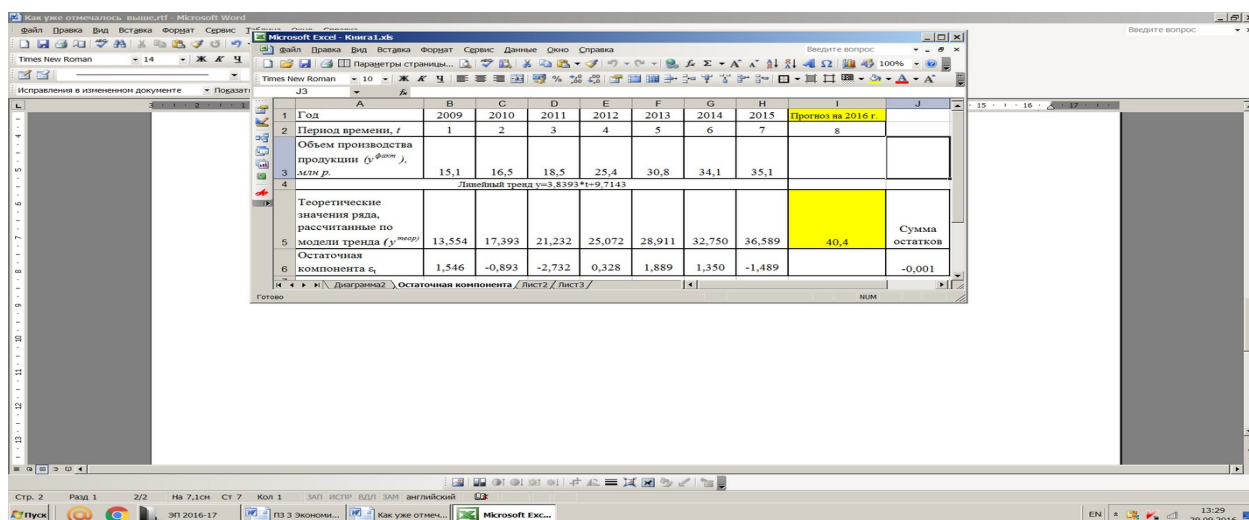
Рисунок 3.5 – Результаты расчета остаточной компоненты
