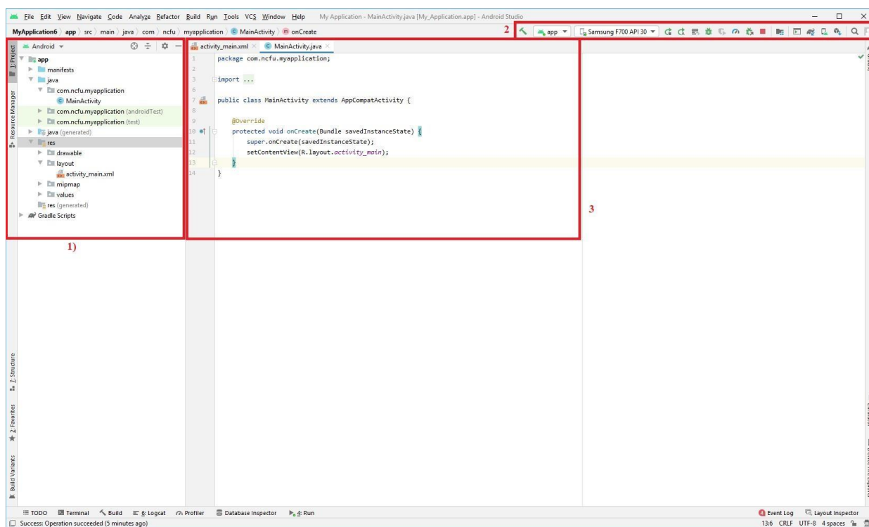
Рисунок 12 – Интерфейс Java
