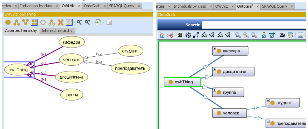
а) OWLViz
