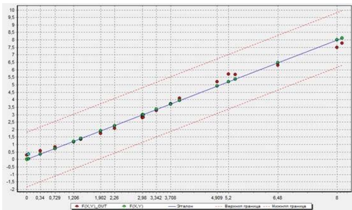
Рис. 2.12. Диаграмма рассеяния
