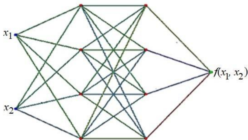
Рис. 2.11. Граф нейросети
