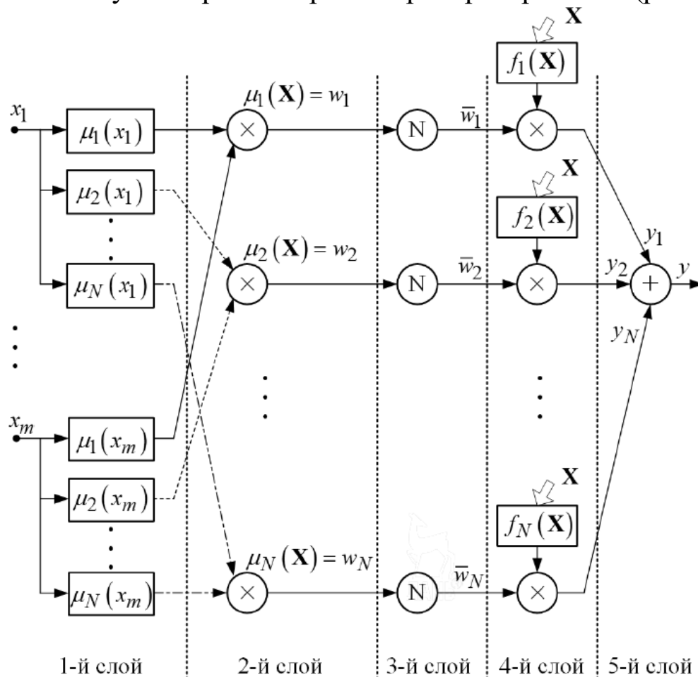
Рис. 4.2. Структура ANFIS-сети
