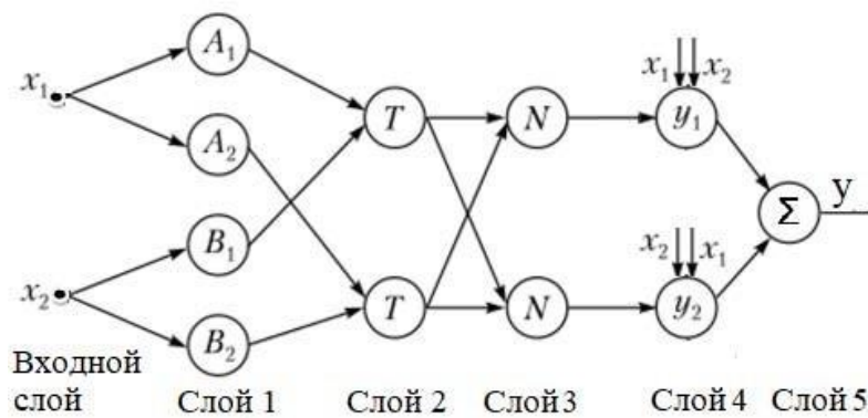
Рис. 4.3. Пример ANFIS-сети
