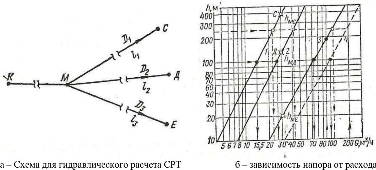
Рисунок 12.2 – Разветвленный трубопровод
