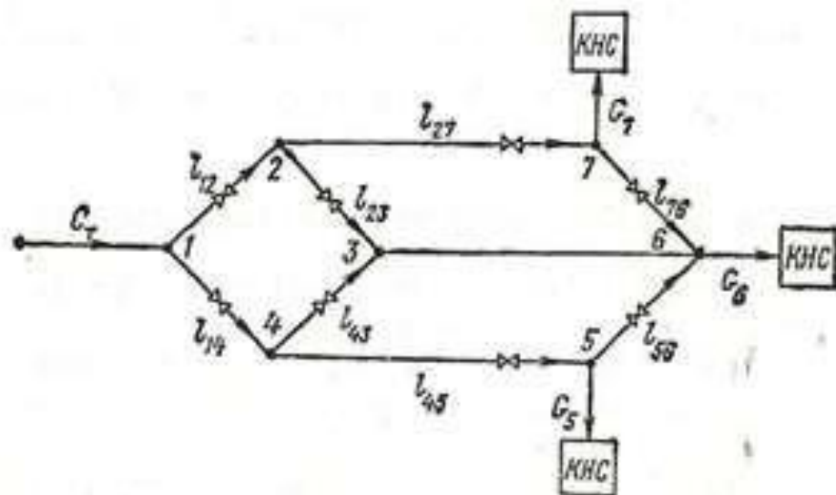
Рисунок 12.1 – Кольцевой трубопровод
