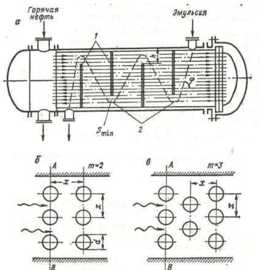
Рисунок 15.2 – Кожухотрубчатый теплообменник:
