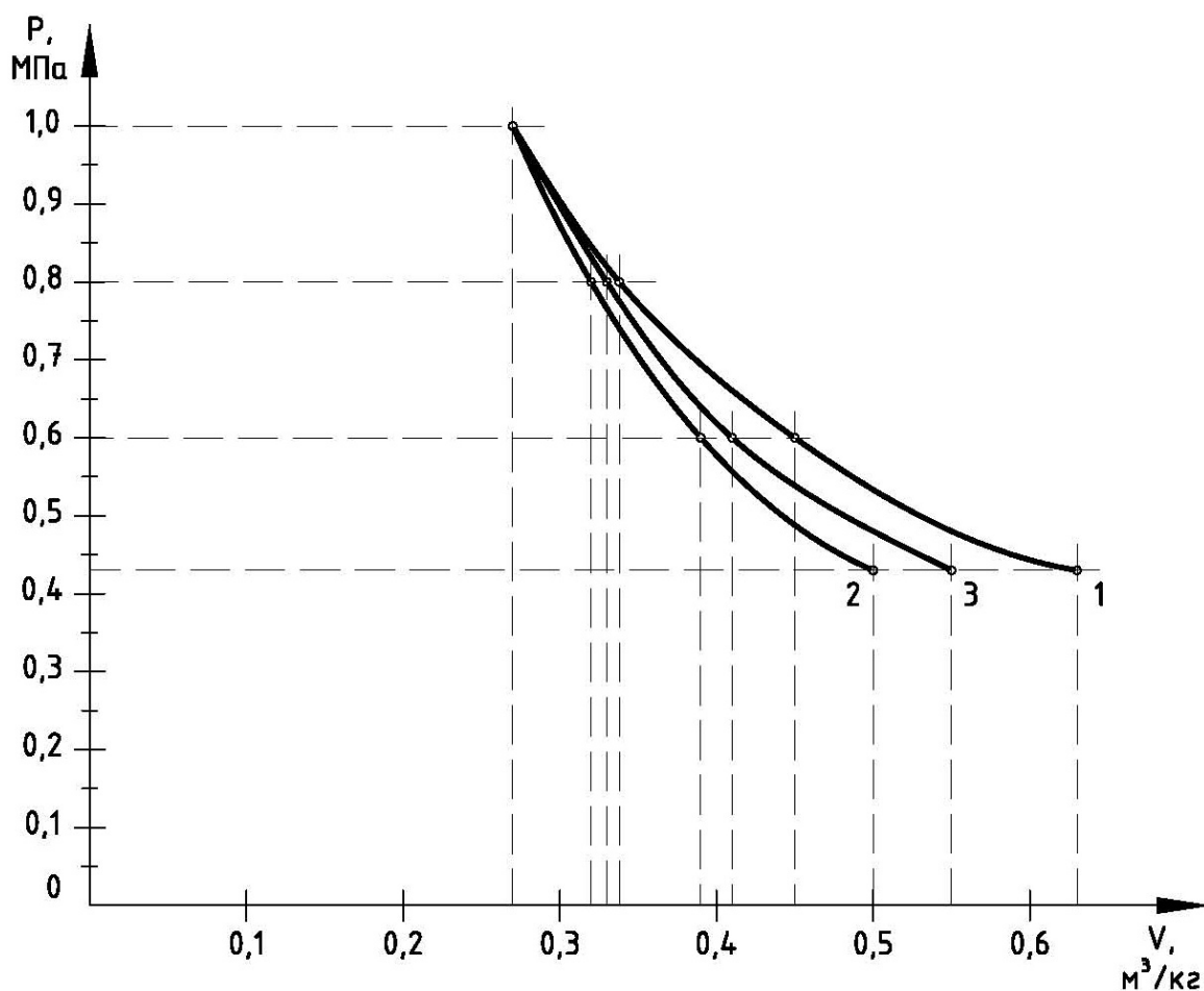
Рисунок 1. P v диаграмма
