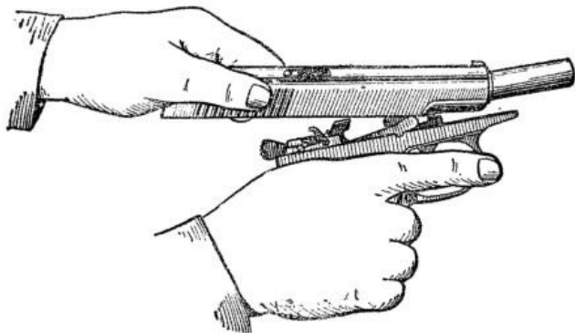
Рис. 7. Присоединение затвора к рамке
