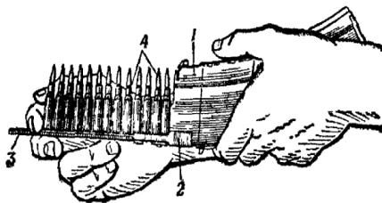
Рис. 63. Снаряжение магазина патронами из обоймы:
