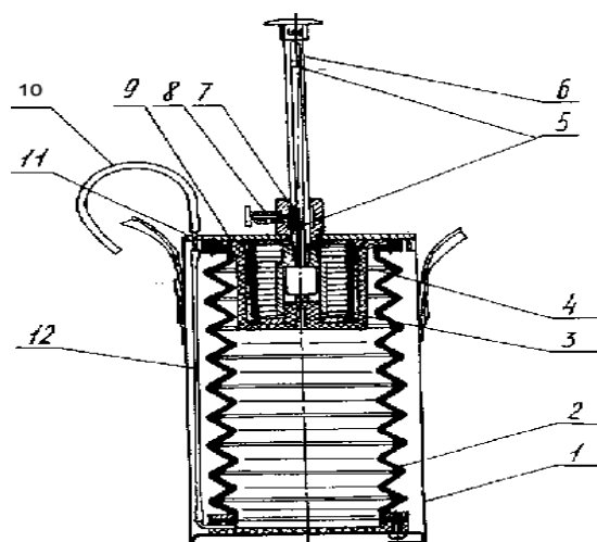
Рис. 12. Газоанализатор УГ-2
