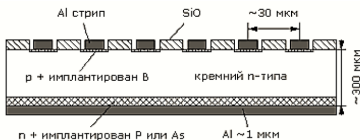
Рисунок 2.5 – Устройство кремниевого микрострипового детектора
