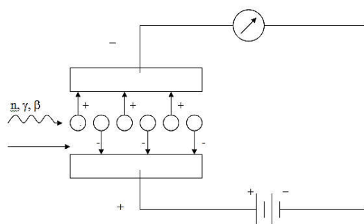
Рисунок 2.3 – Принципиальная схема работы ионизационной камеры
