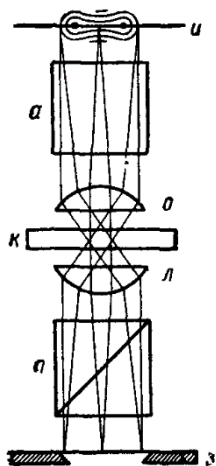
Рис. 34. Схема наблюдения интерференционной фигуры способом Лазо:
