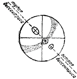
Рис. 37. Интерференционная фигура двuosного минерала на разрезе, перпендикулярном к оптической оси.
