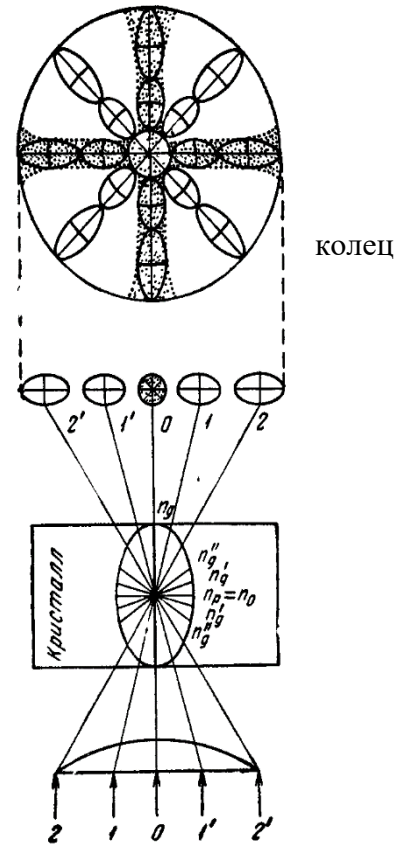
Рис. 35. Схема получения интерференционной фигуры одноосного оптически положительного минерала на разрезе, перпендикулярном к оптической оси.
