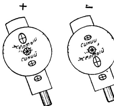
Рис. 39 Определение оптического знака двусосного минерала в разрезе, перпендикулярном к оптической оси с помощью кварцевой пластинки.
