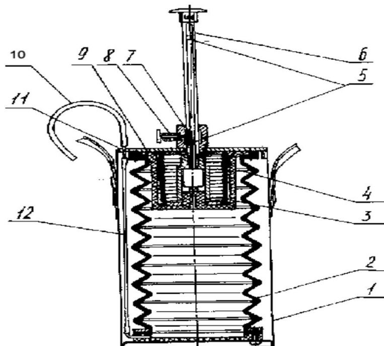
Рис. 12. Газоанализатор УГ-2
