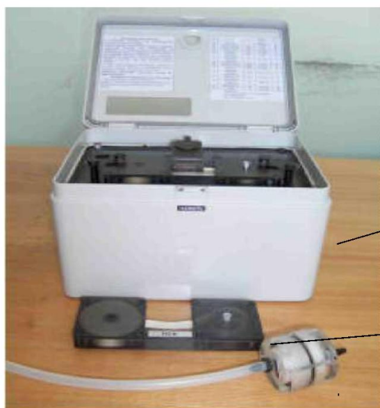
Рисунок 3.2 – Общий вид газоанализатора ГАНК-4
