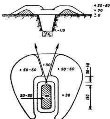
Одиночный окоп для стрельбы из автомата стоя
