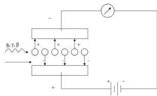
Рисунок 2.3 – Принципиальная схема работы ионизационной камеры
