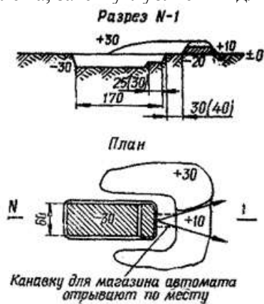
Одиночный окоп для стрельбы из автомата лежа
