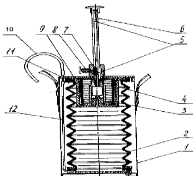
Рис. 12. Газоанализатор УГ-2
