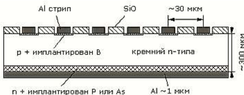
Рисунок 2.5 – Устройство кремниевого микрострипового детектора
