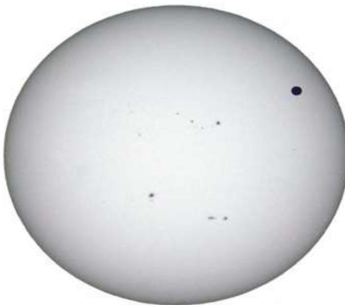
Рис. Фотография прохождения Венеры по диску Солнца 6 июня 2012 года
