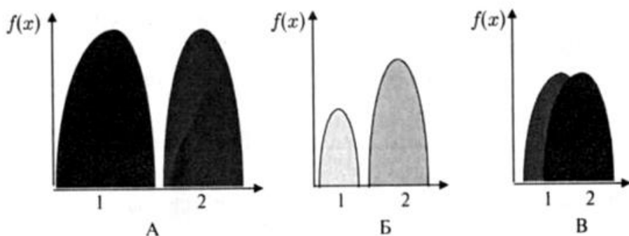
Рис. 5.6. Функция отклика (выживаемости) двух разных организмов в зависимости от температуры
