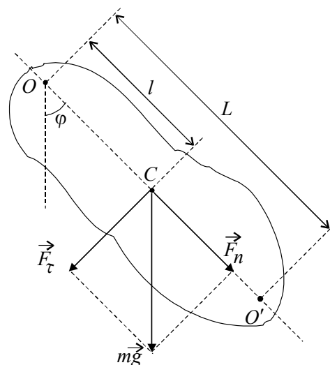
Рис. 1. Физический маятник
