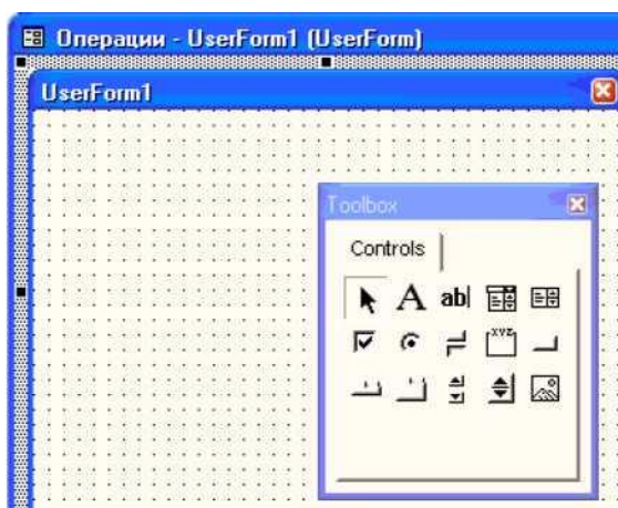
Рис. 12. Новая форма
