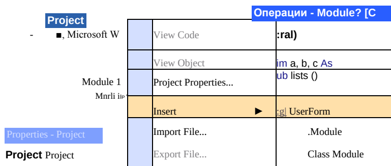
Рис. 11. Добавление формы
