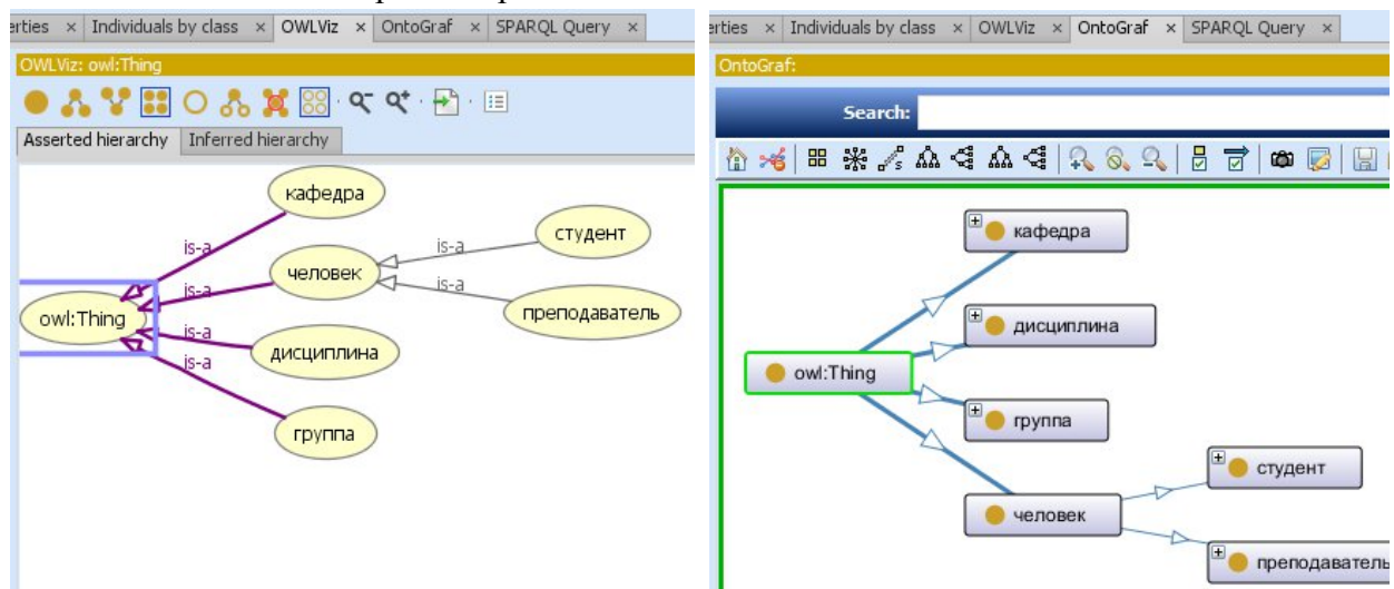
а) OWLViz
