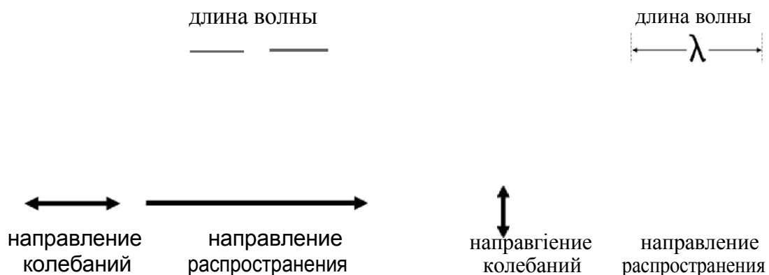
Рисунок 4.1 — Продольная и поперечная волны
