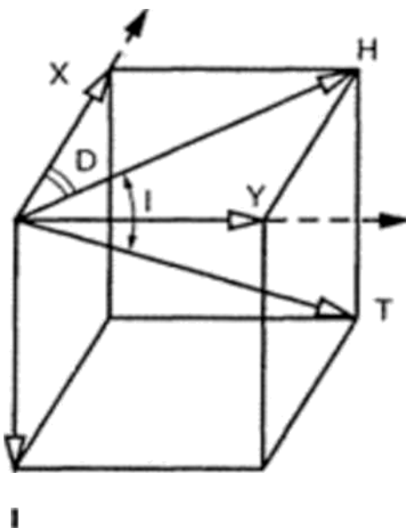
Рис. 7.1 — Составляющие магнитного поля Земли
