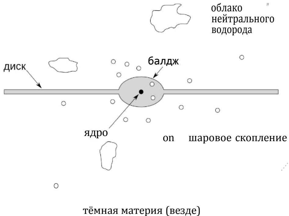
Рис. 1.9 — Схема спиральной галактики
