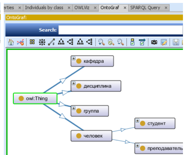
б) OntoGraf
