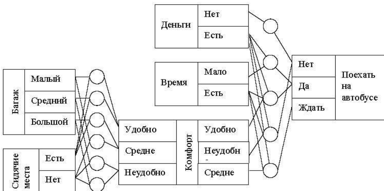
Рисунок 1.5 – Дерево правил
