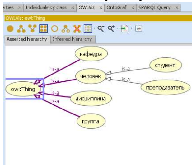
а) OWLViz
