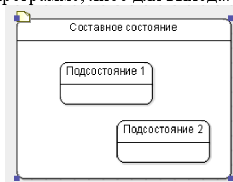
Рисунок 7.6 – Составное состояние
