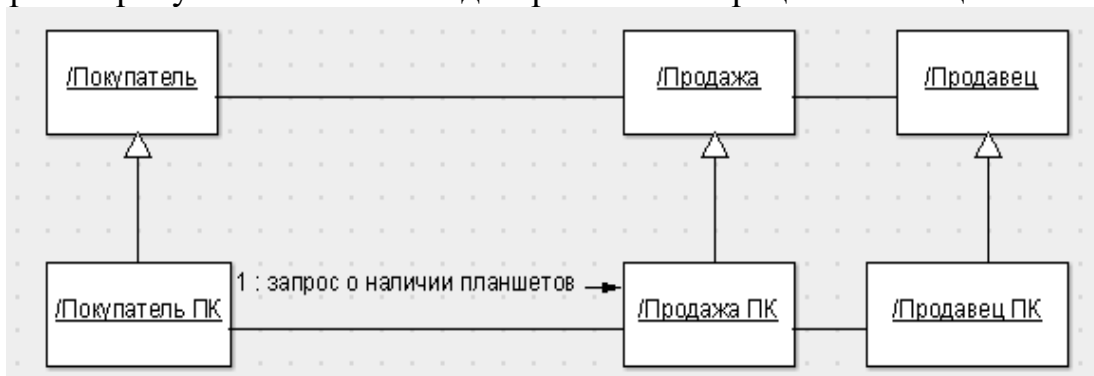
Рисунок 6.4 – Диаграмма кооперации
