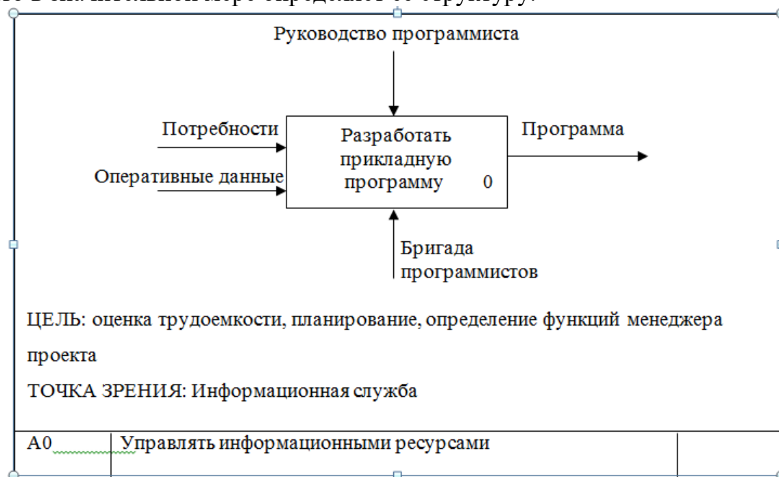
Рисунок 17.4 – Контекстная диаграмма
