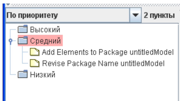
Рисунок 2.5 – Панель «To-do»
