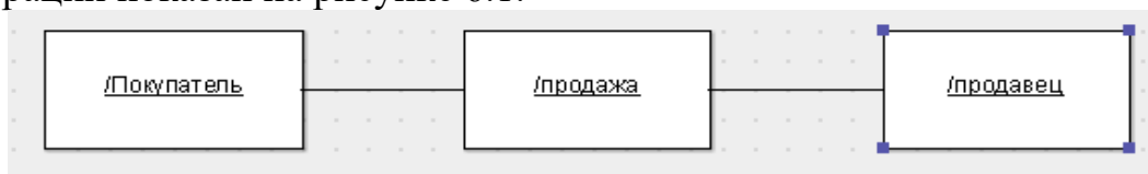
Рисунок 6.1 – Диаграмма кооперации
