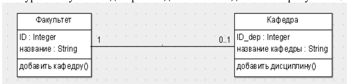
Рисунок 4.6 – Диаграмма классов
