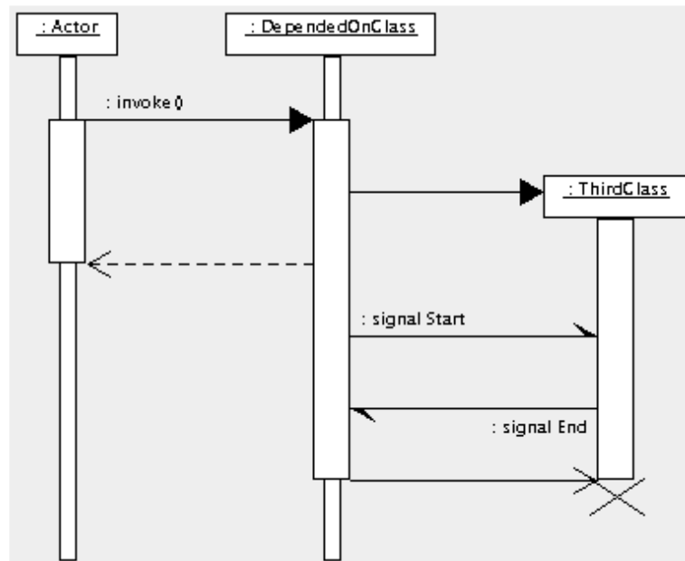
Рисунок 5.1 – Диаграмма последовательности
