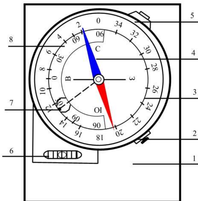
Рисунок 8 – Горный компас (1 – металлическая пластинка, 2 – стопорный винт, 3 – лимб, 4 – магнитная стрелка, 5 – стопор отвеса, 6 – уровень, 7 –
