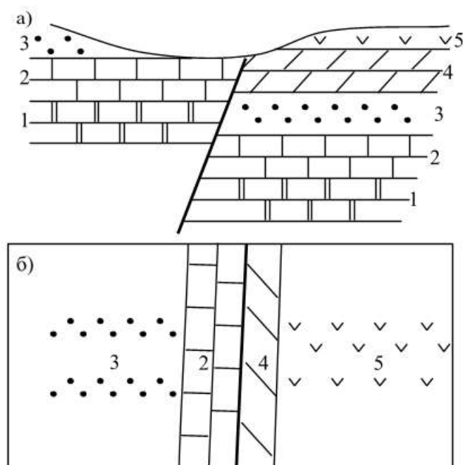
Рисунок 16 – Разрывное залегание пород (а – разрез, б – карта)
