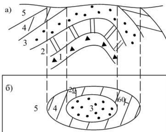
Рисунок 14 – Складчатое залегание пород (а – разрез, б – карта)
