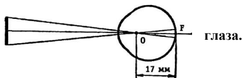
Рис. 6. Расположение узловой точки и заднего фокуса глаза.
