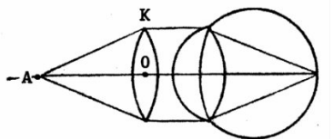
Рис. 7. Схема, поясняющая расчет силы аккомодации.
