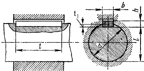
Рисунок 14 – Расчетная схема
