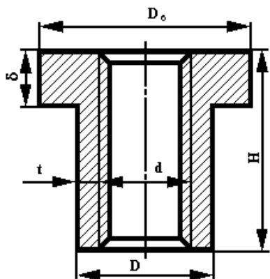
Рисунок 40 – Расчетная схема
