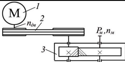
Схема 1. Редуктор цилиндрический
