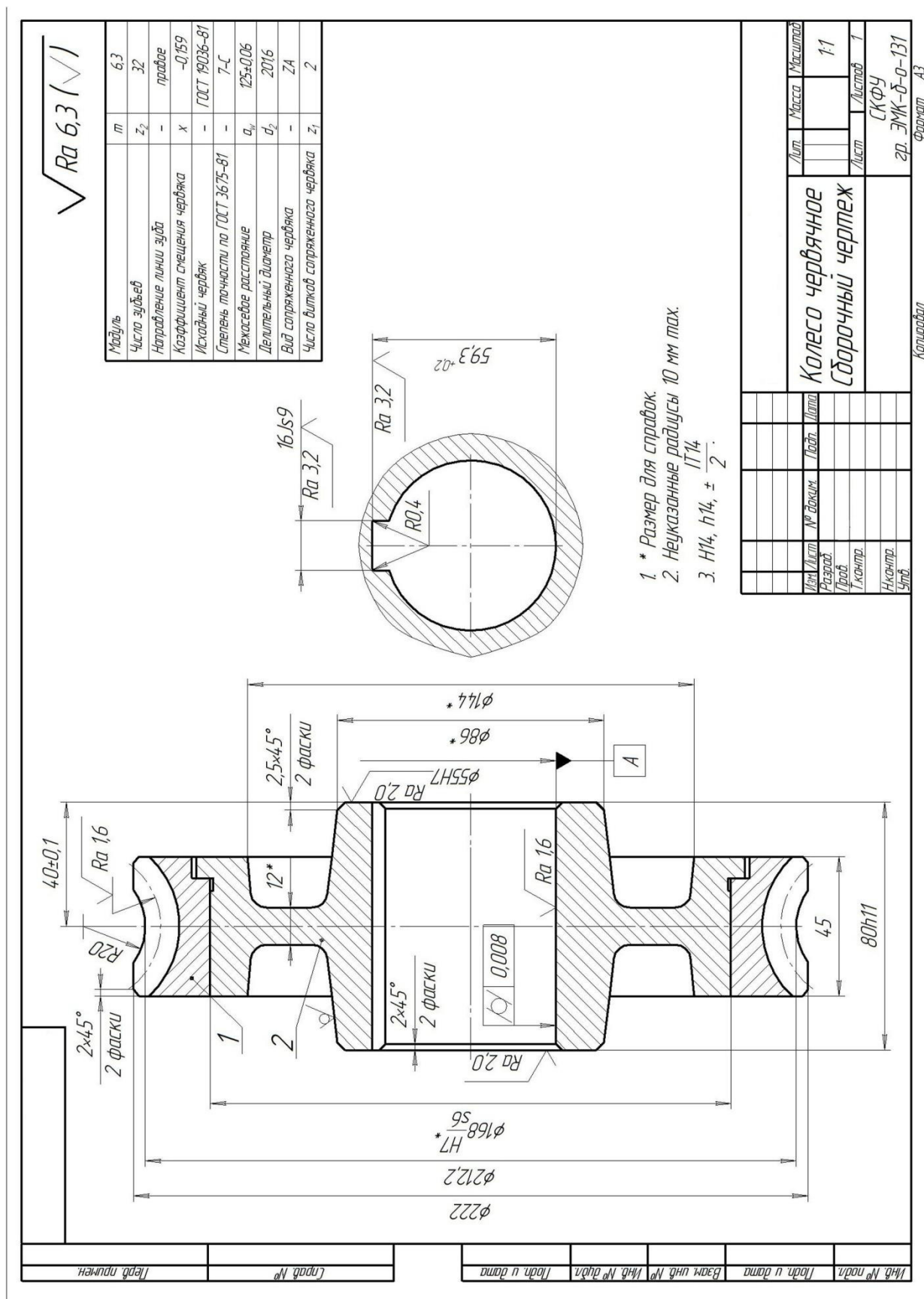
Рисунок 6 – Рабочий чертеж червячного колеса
