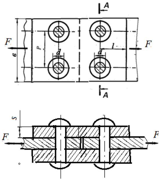
Рисунок 2-Заклепочный шов
