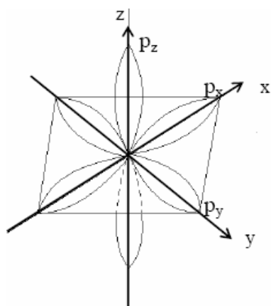
Рис. 5. Расположение p -орбиталей металла в квадратном комплексе dsp^2 -орбитали.
