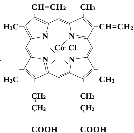
Кобальтовый комплекс протопорфирина-IX
