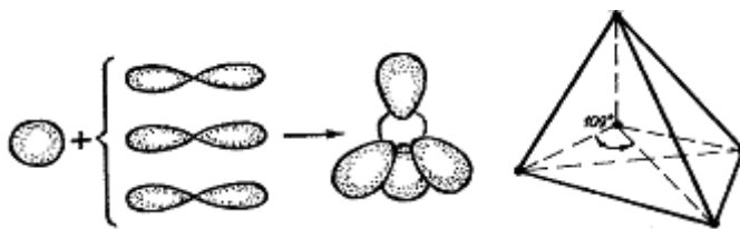
Рис.4. sp^3 -гибридизация атомных орбиталей
