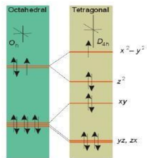
Рис. 11. Расщепление d -орбиталей иона \text{Cu}^{2+} ( d^9 ) [http://www.chem.msu.ru/rus/teaching/shevelkov2.pdf]
