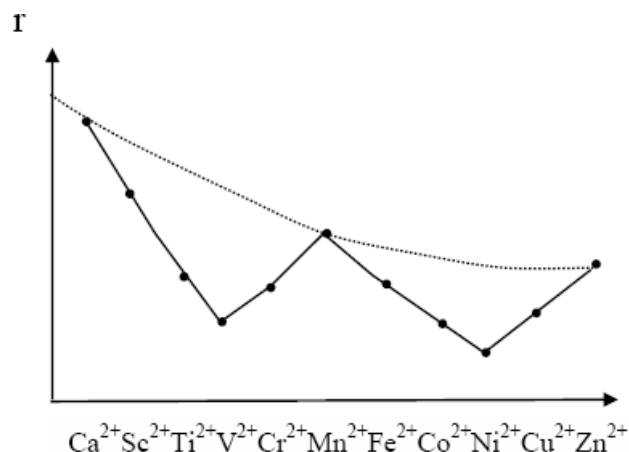
Рис. 10. Относительные значения ионных радиусов
