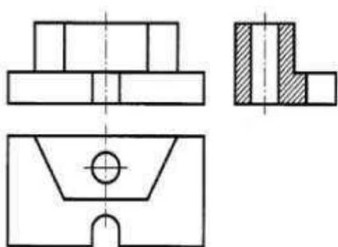
Рисунок 1.4—Профильный разрез
