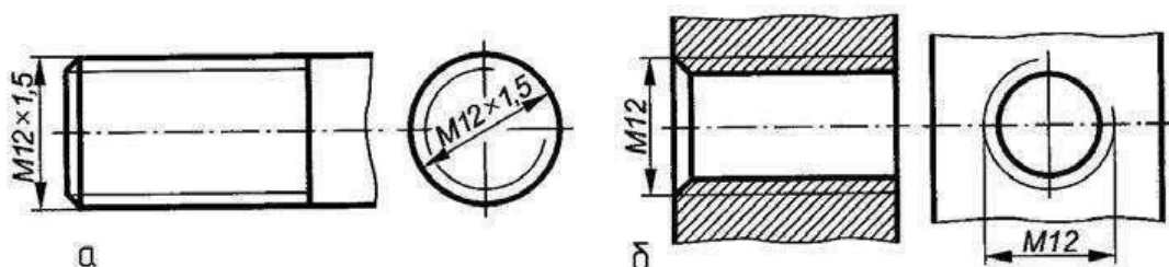
Рисунок 3.5 – Метрическая резьба
