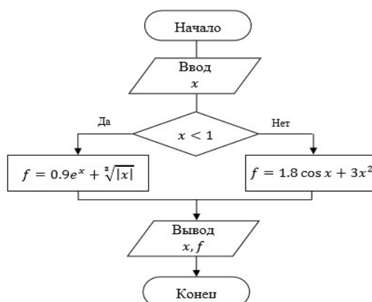
Блок-схема алгоритма
