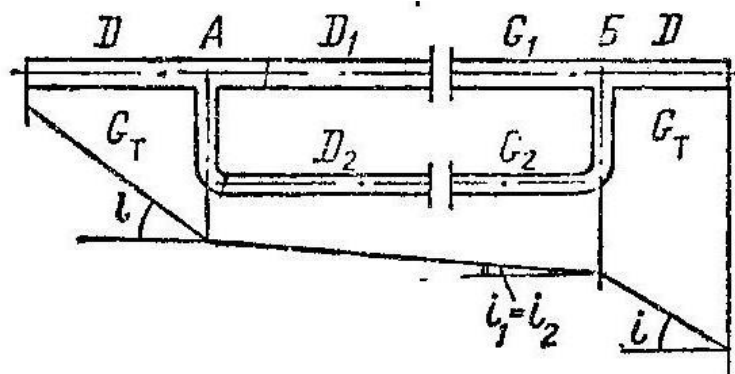
Рисунок 6.3 – Коллектор с параллельным участком
