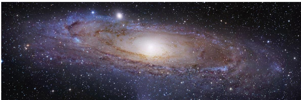
Рис. 1.3 – Спиральная галактика
