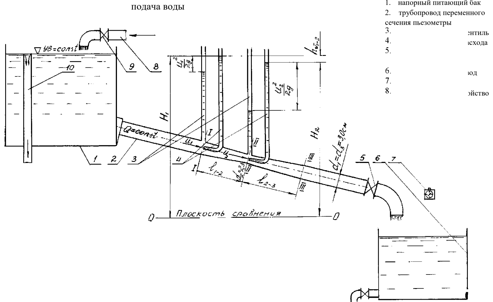
Рисунок 6.1 . Схема установки для экспериментальной иллюстрации уравнения Д. Бернулли
