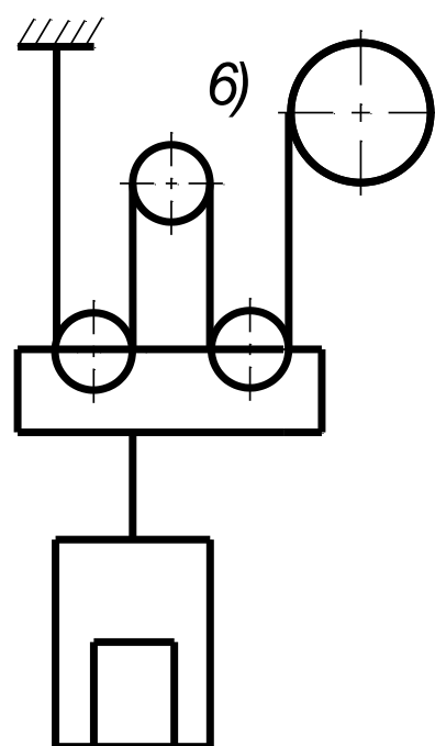
1 – блок; 2 – барабан лебедки; 3 – грузовая площадка; 4 – груз Рисунок 3.1 - Схема запасовки каната в полиспастах
