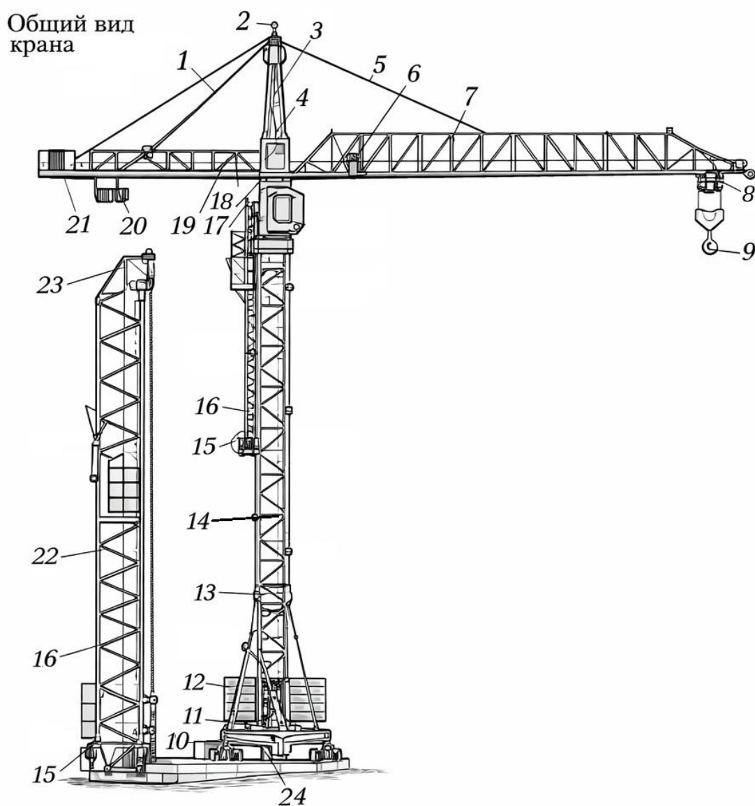
Рисунок 4.1 - Башенный кран
