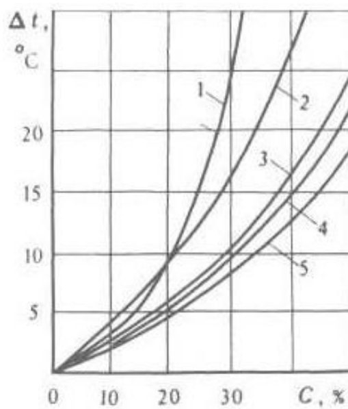
Рисунок 3.3 – Зависимости снижения температуры образования гидратов от массового содержания различных химических агентов: 1 – \text{CaCl}_2 ; 2 – \text{CH}_3\text{OH} ; 3 – триэтиленгликоль; 4 – диэтиленгликоль (ДЭГ); 5 — этиленгликоль.
