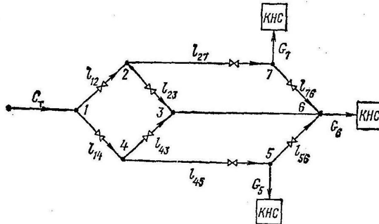
Рисунок 6.2 – Схема сложного кольцевого водовода
