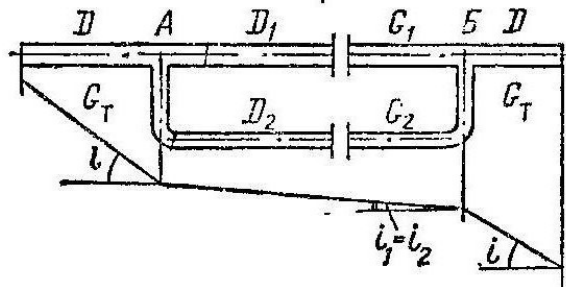
Рисунок 6.3 – Коллектор с параллельным участком
