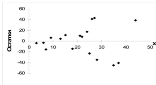
Рисунок 8 – Колебания остатков
