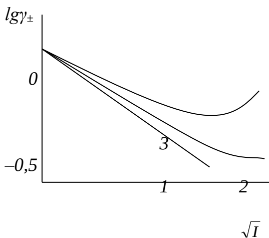
Рисунок 12.1 – Зависимость \lg \gamma_{\pm} от \sqrt{I} для LiCl: 1 – предельный закон (8.15), 2 – по уравнению второго приближения (12.16), 3 – экспериментальная кривая
