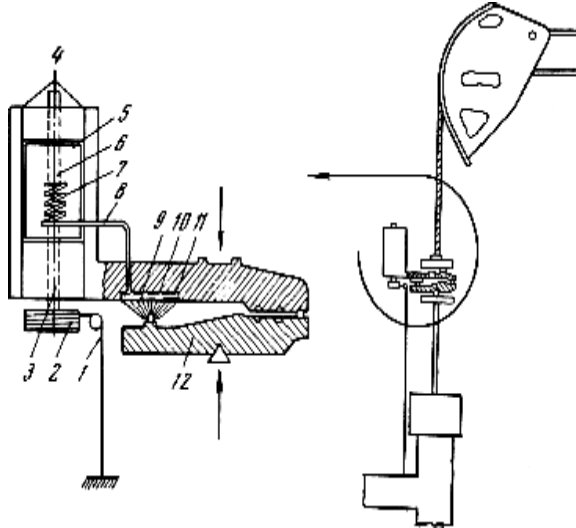
Рисунок 1 - Динамограф ГДМ-3
